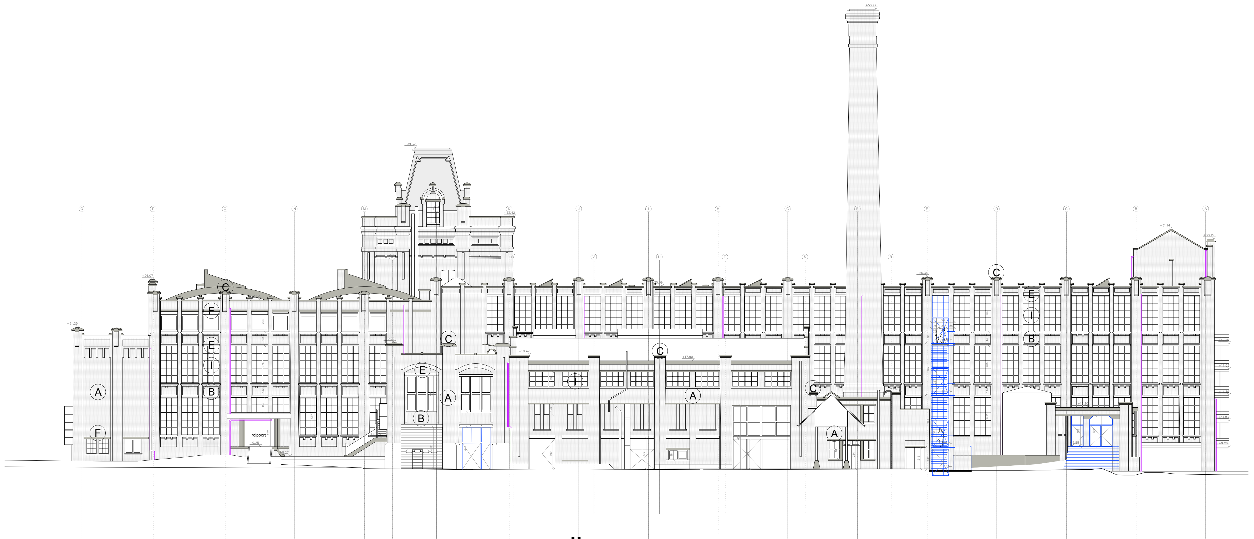
RECHTERGEVEL (OOST) - NIEUWE TOESTAND - 1/200 -
