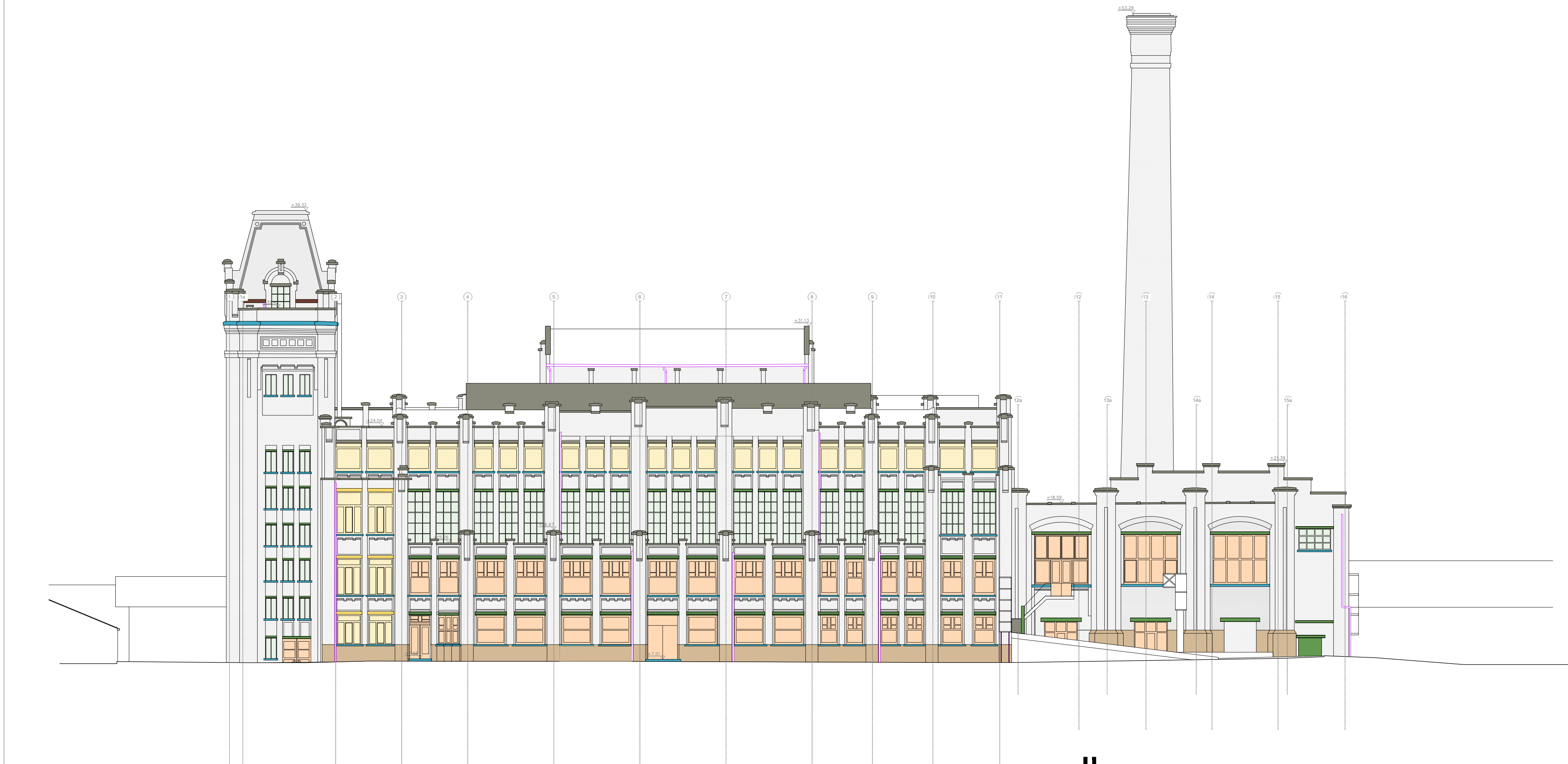
VOORGEVEL (WEST) - BESTAANDE TOESTAND - 1/200 -
