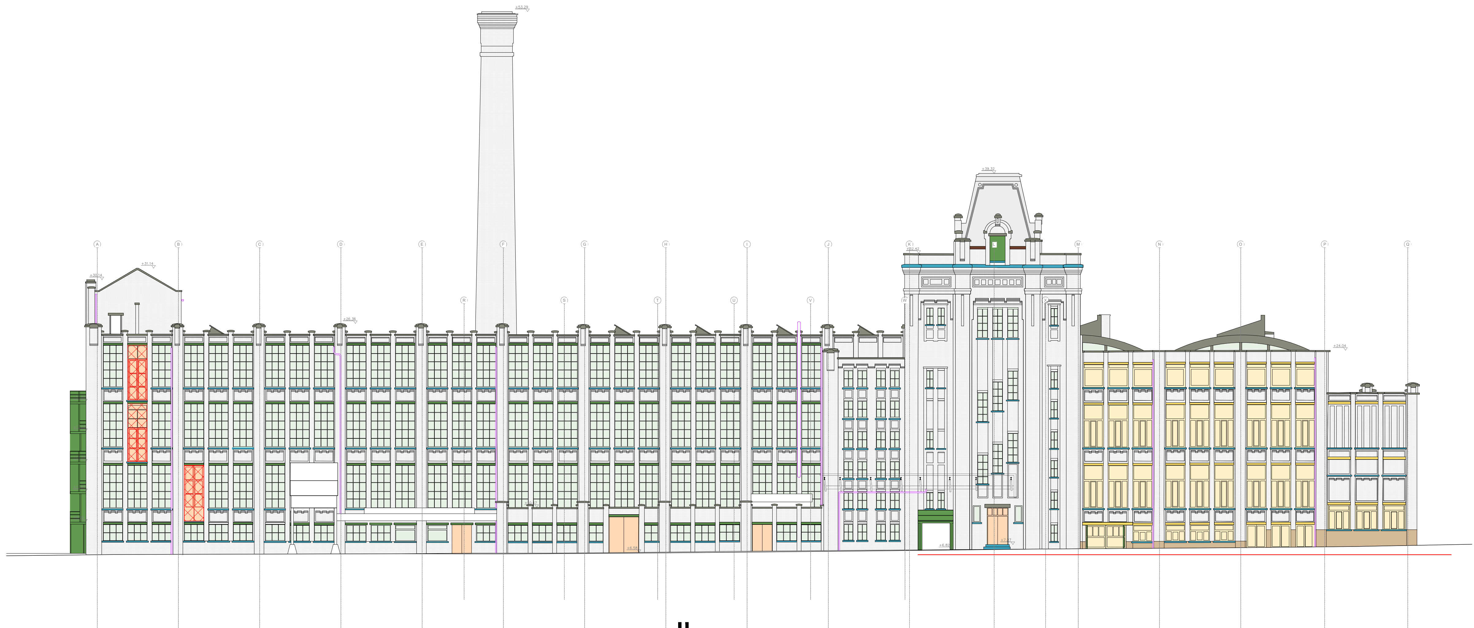
LINKERGEVEL (WEST) - BESTAANDE TOESTAND - 1/200 -
