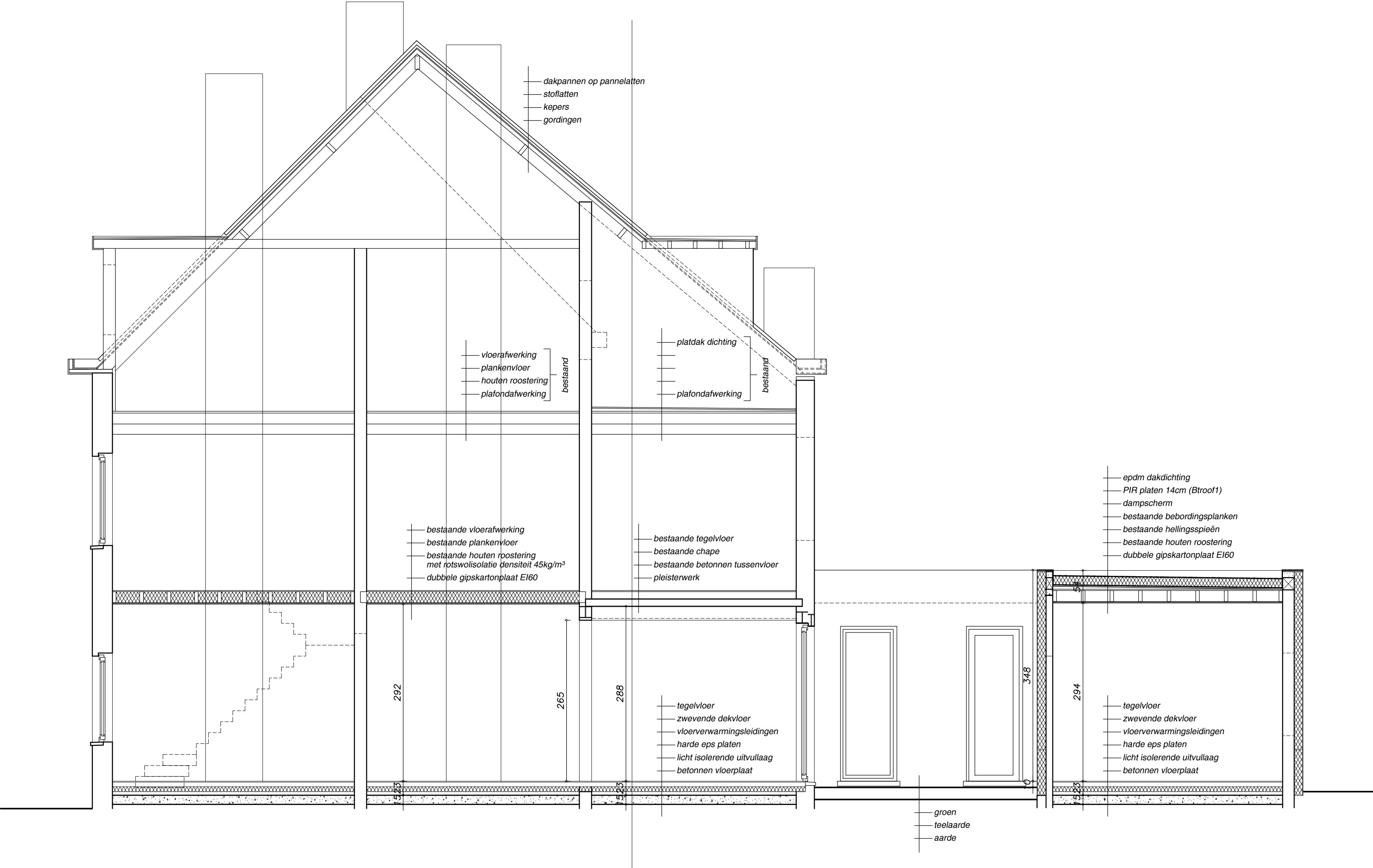
LANGSSNEDE AA nieuw 1/50 0 2.5m
