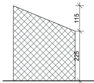
VOORGEVEL
