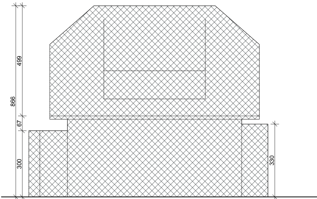
LINKERGEVEL
