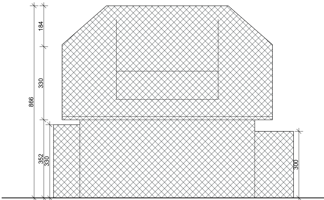
RECHTERGEVEL
