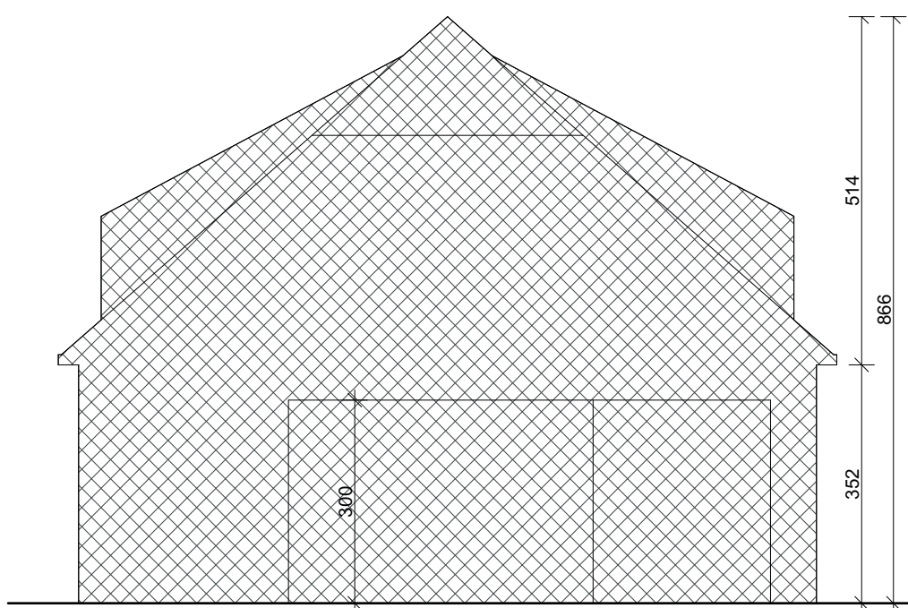
ACHTERGEVEL
