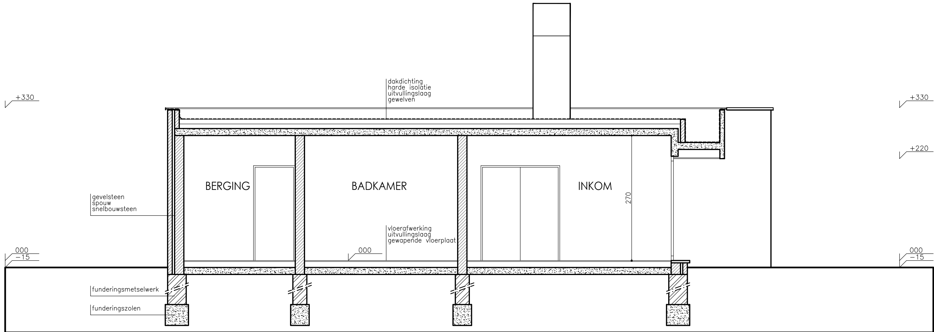
DOORSNEDE AB
