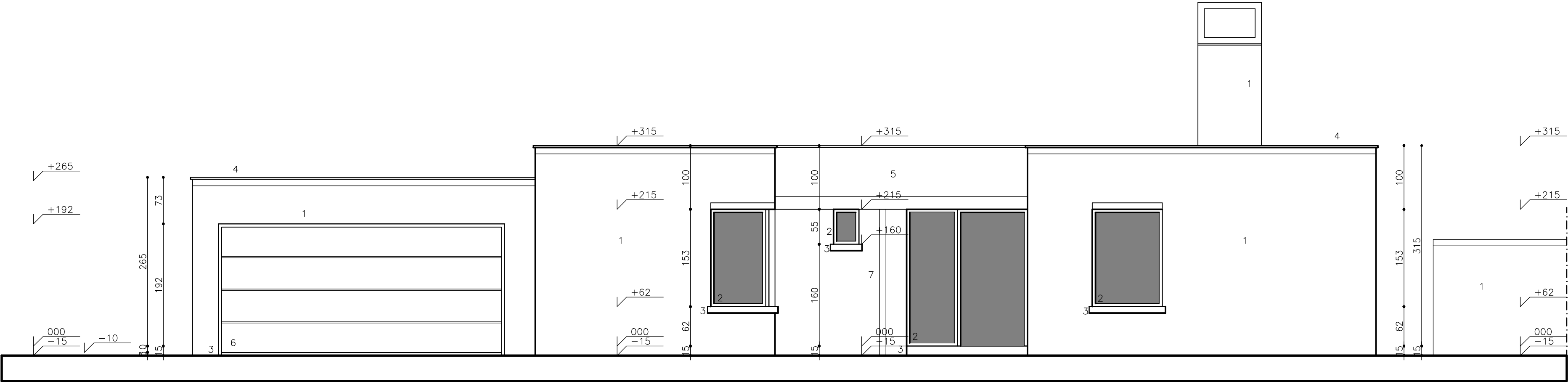
ZIJGEVEL LINKS
