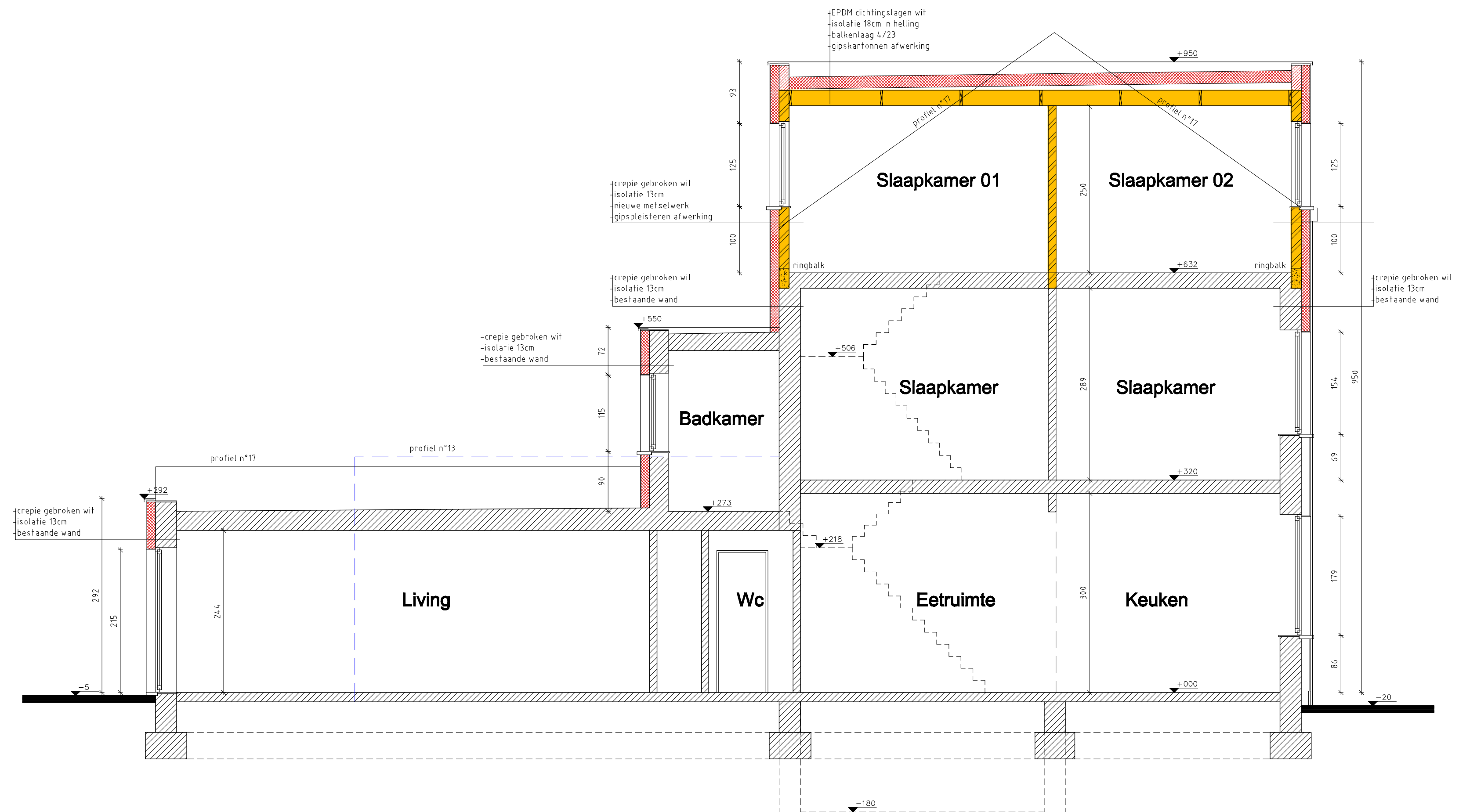
doorsnede AA' nieuwe toestand 1/50
