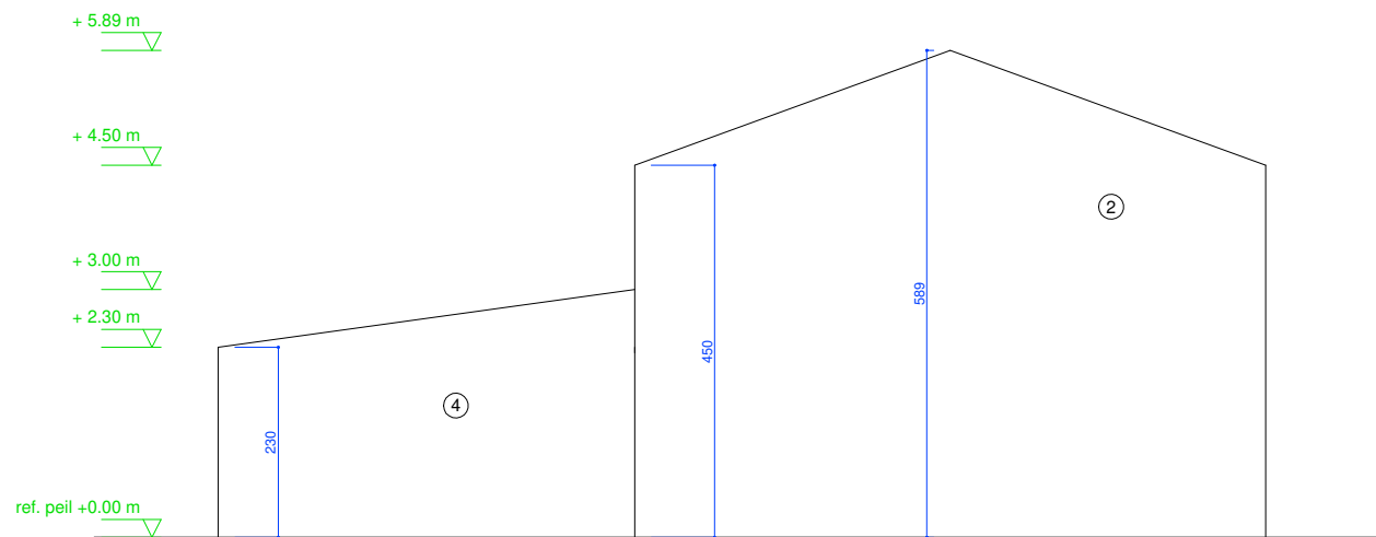
ZIJGEVEL LINKS loods met garages
