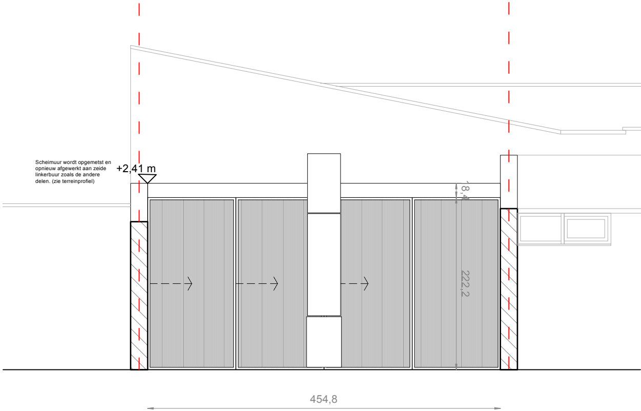
GEVELAANZICHT TUINBERGING Nieuwe toestand 1/50
