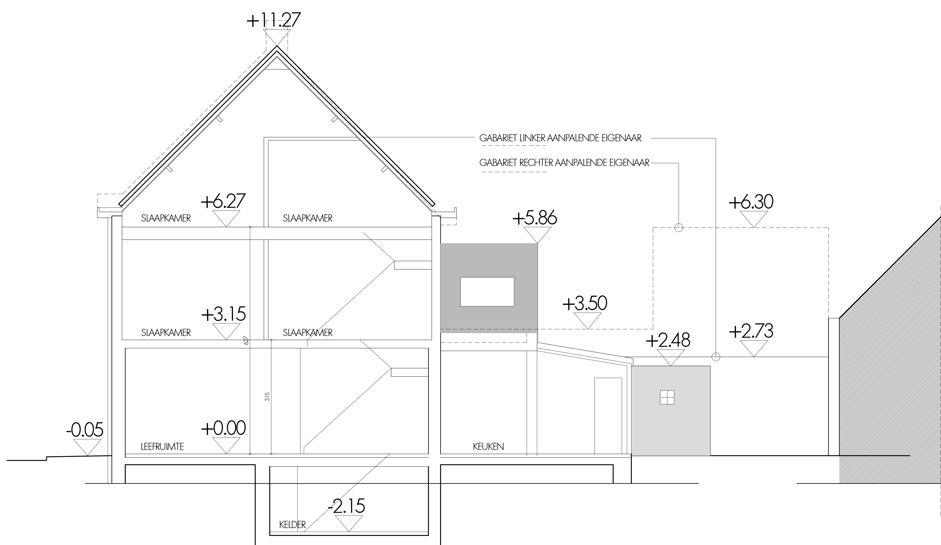
PROFIELDOORSNEDE 1 BESTAANDE TOESTAND
