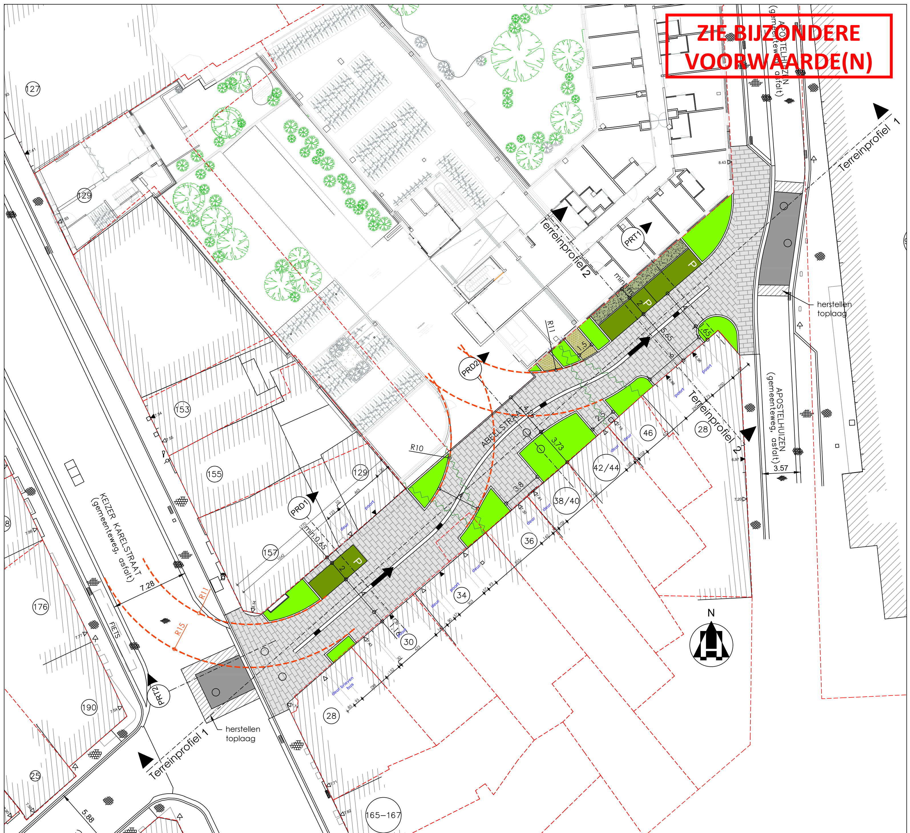
GRONDPLAN - nieuwe toestand
