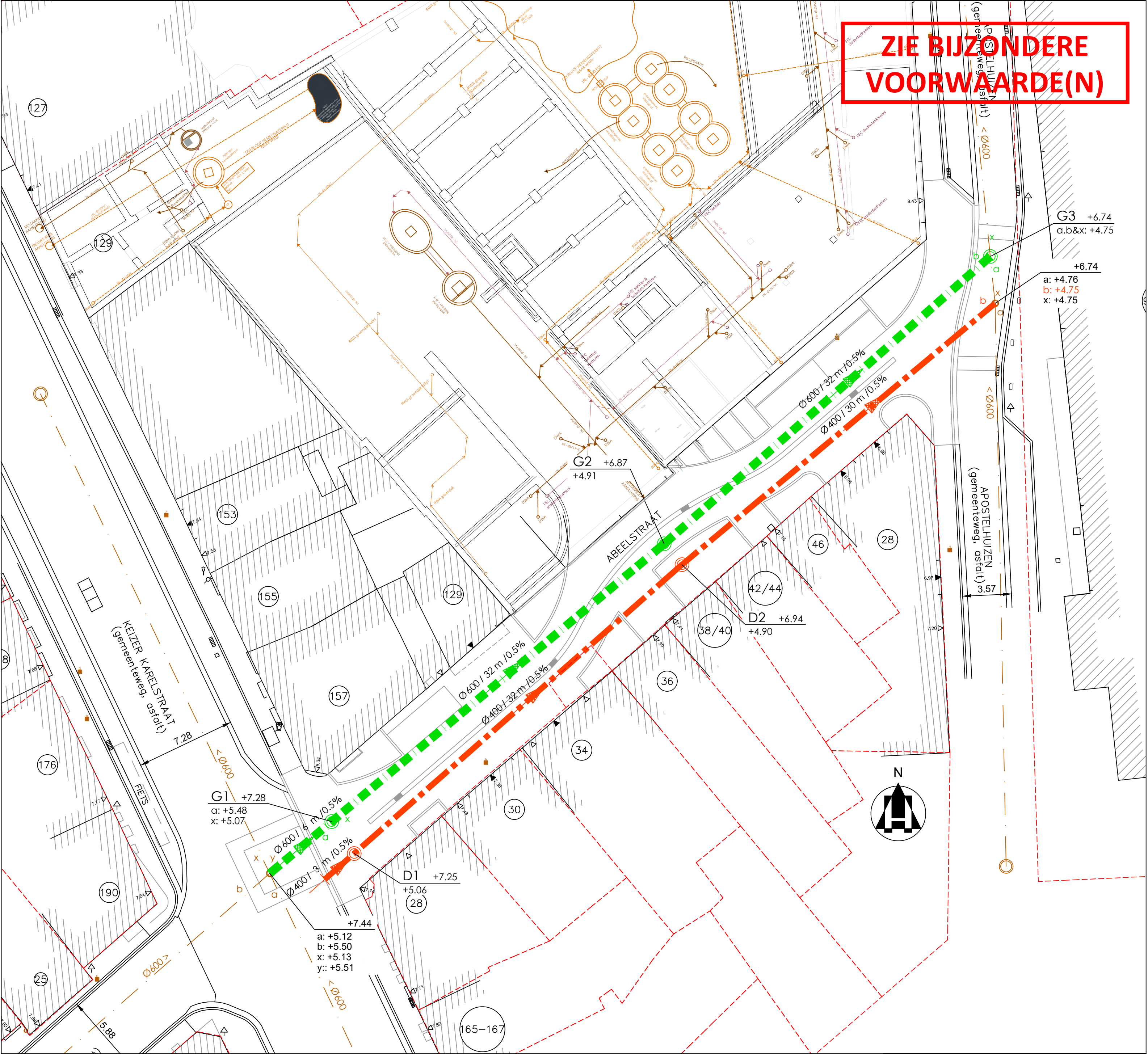
GRONDPLAN - riolering
