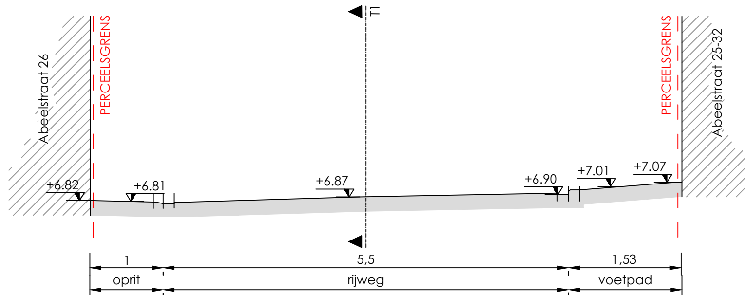
Dwarsprofiel 2
