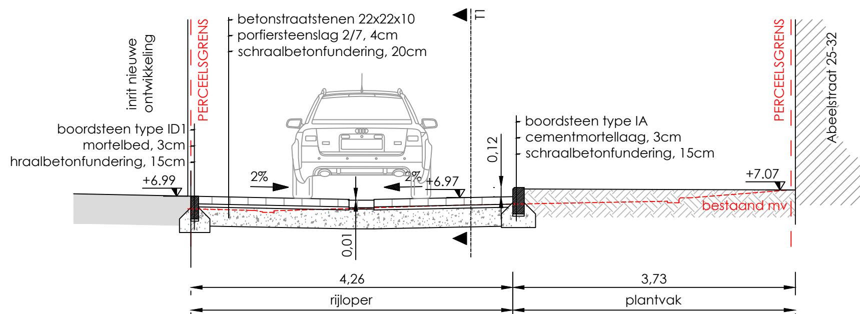
Dwarsprofiel 2
