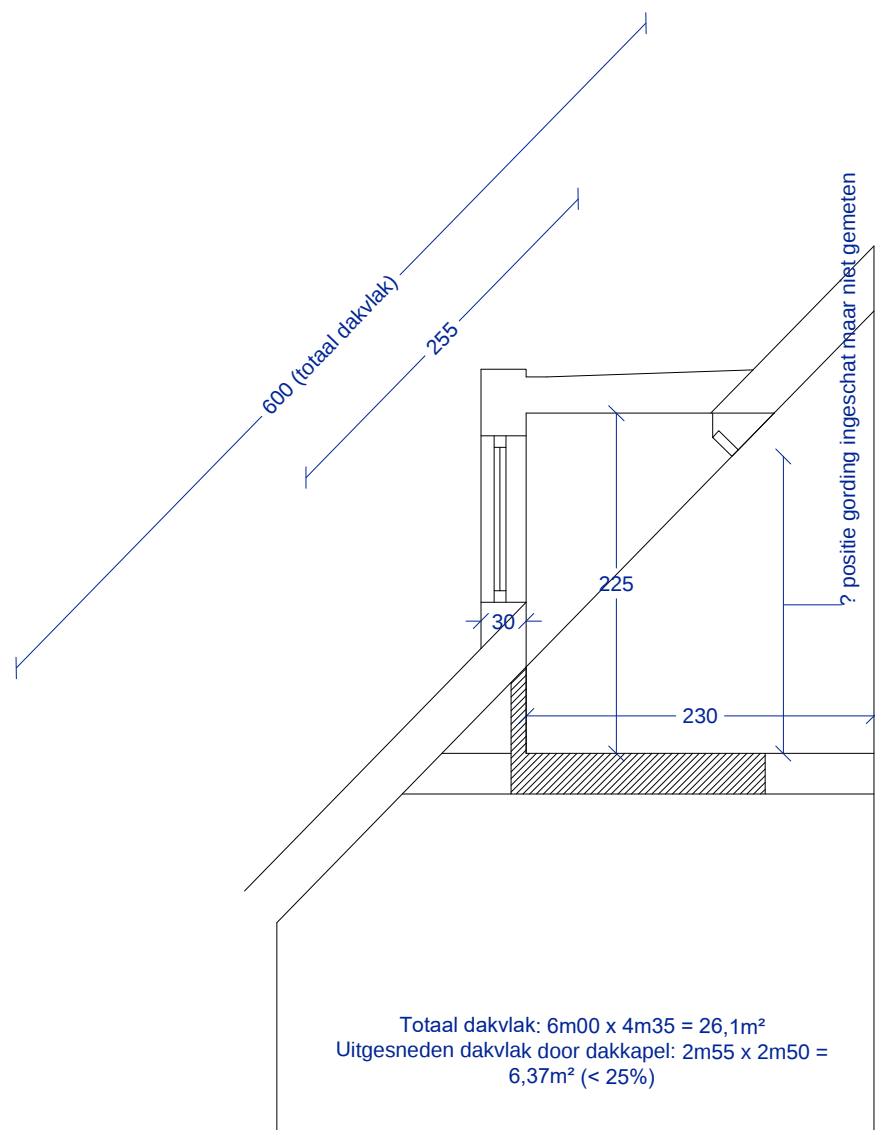
doorsede wooneenheid 49C
