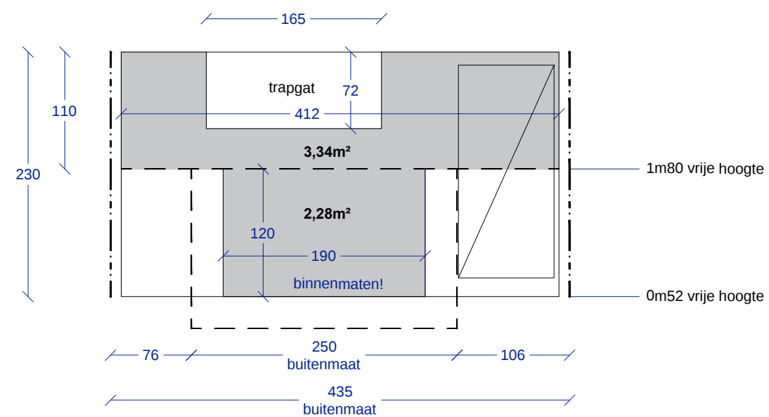
Grondplan mezanine, wooneenheid 49C
