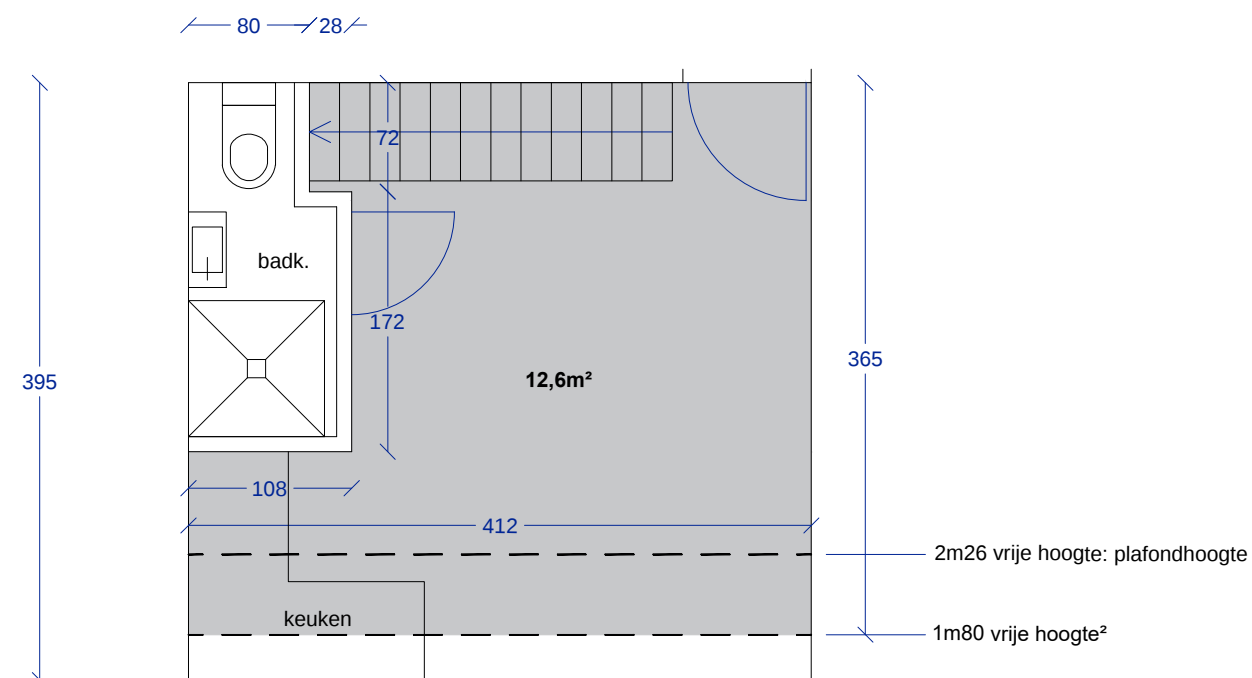
Grondplan +2, wooneenheid 49C
