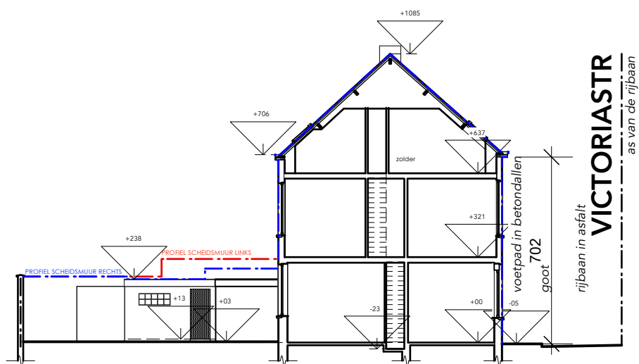
TERREINPROFIEL (1:200)
