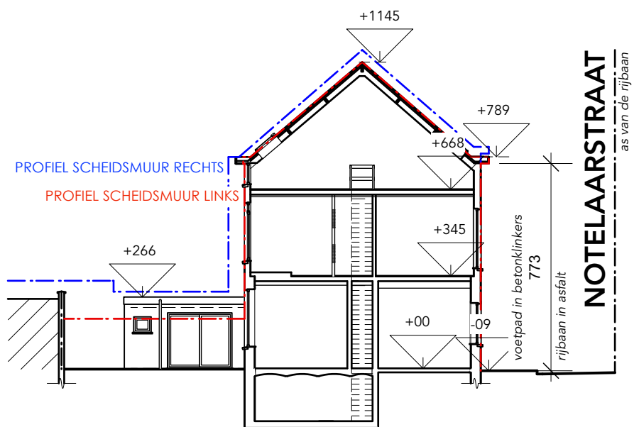
TERREINPROFIEL (1:200)
