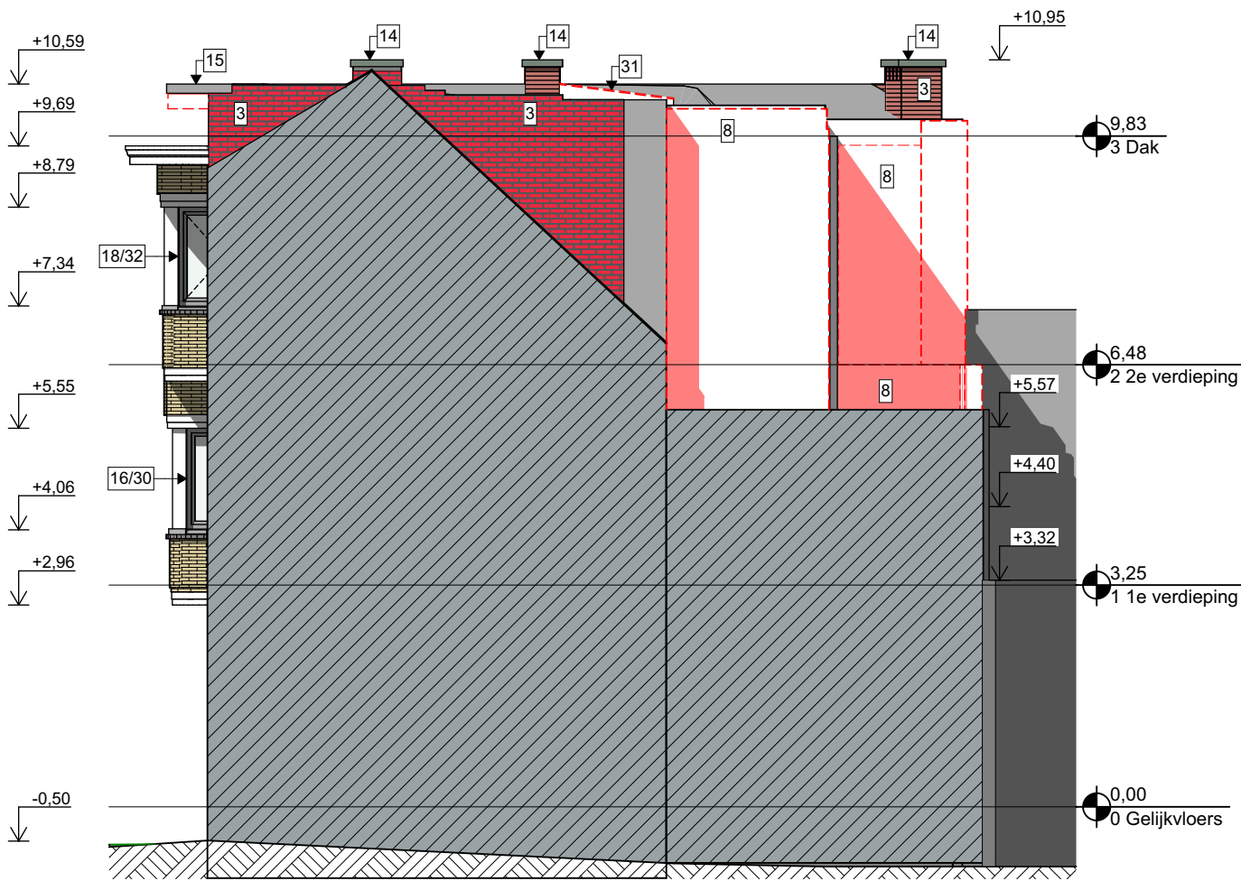
RG Zijgevel Rechts 1:100
