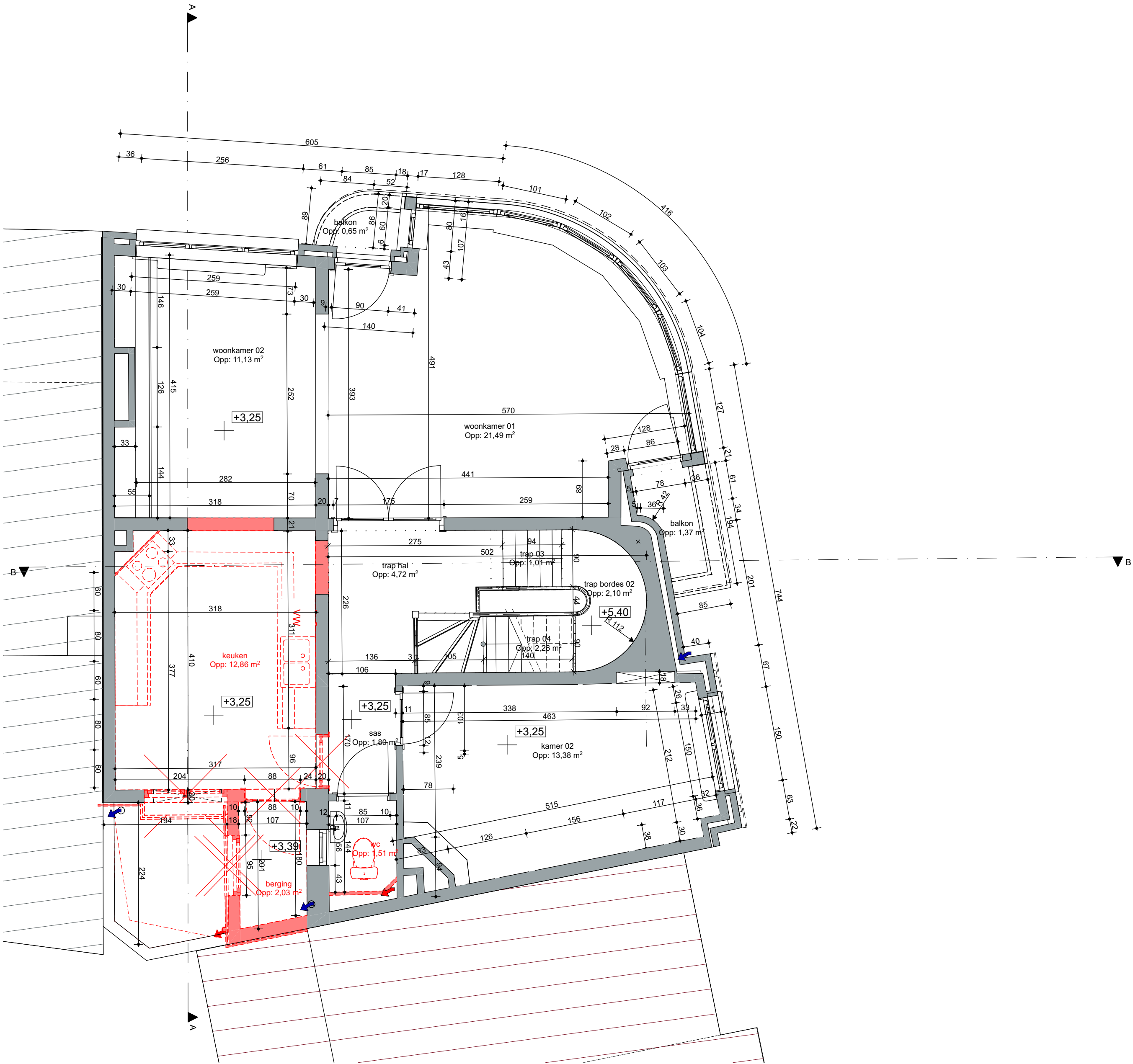
1. 1e verdieping 1:50
