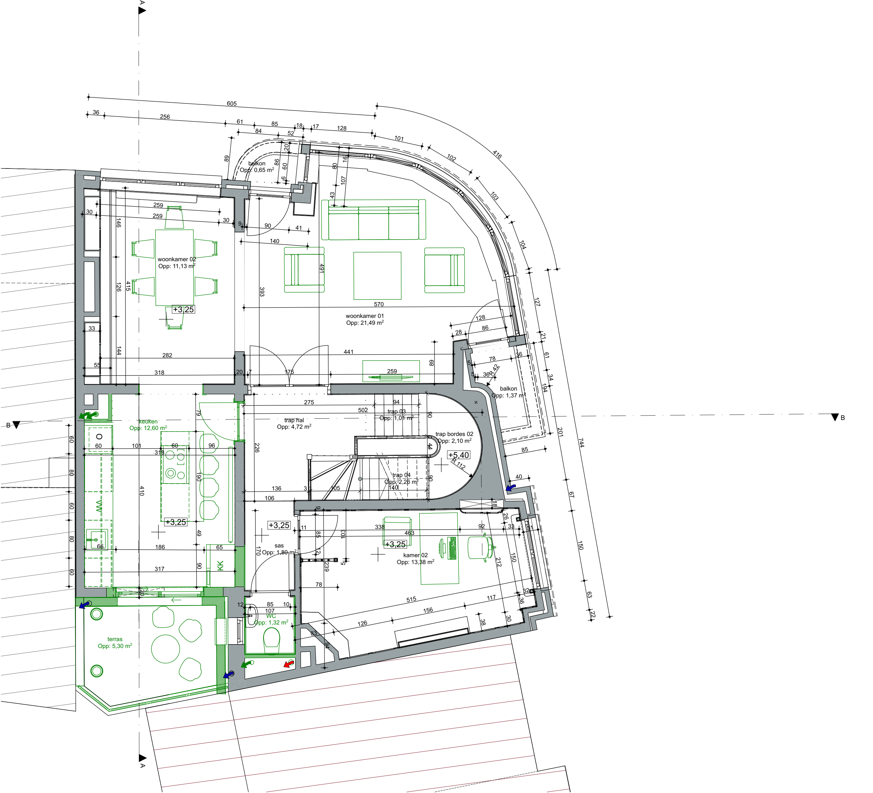
1. 1e verdieping 1:50
