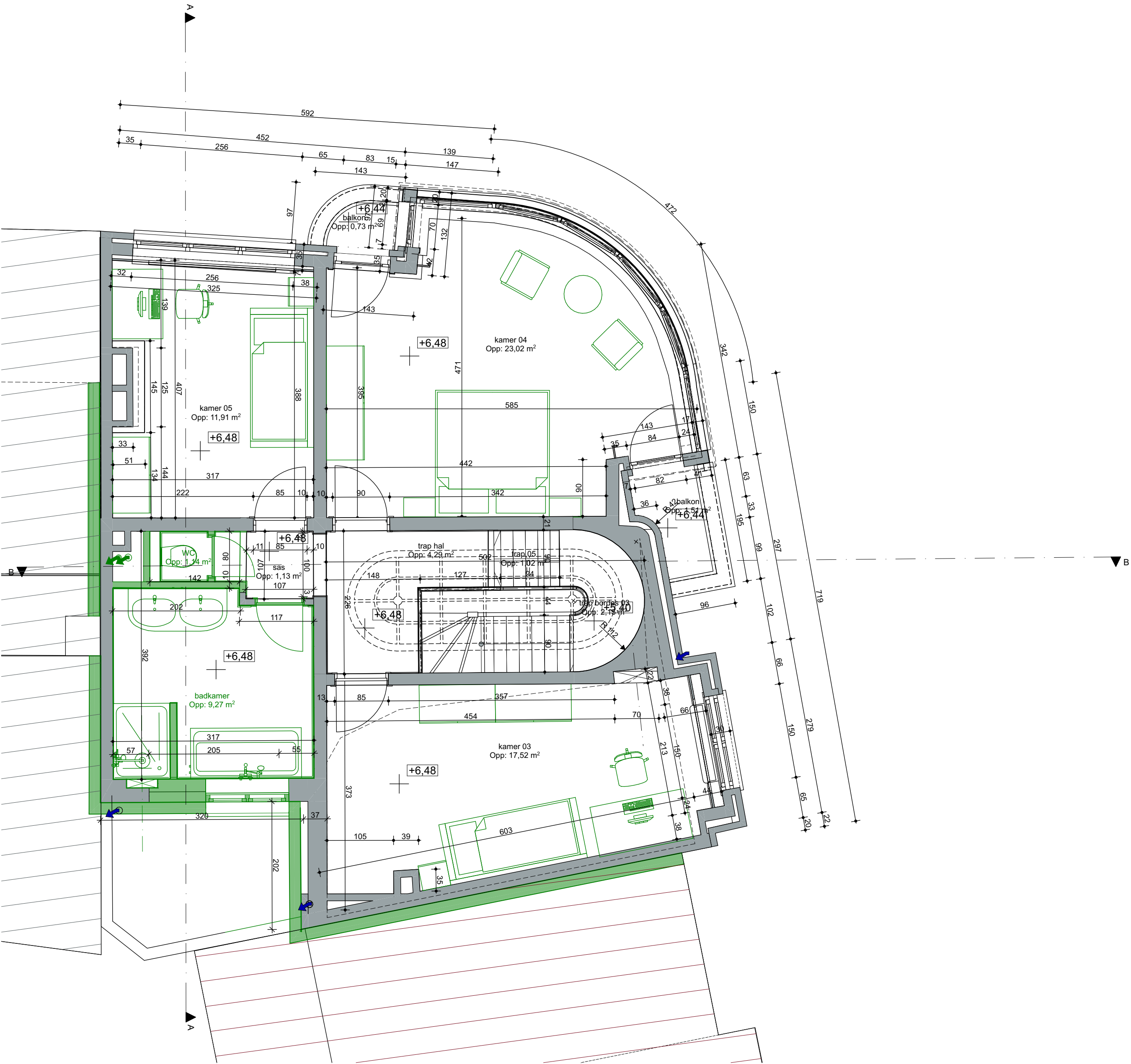
2. 2e verdieping 1:50
