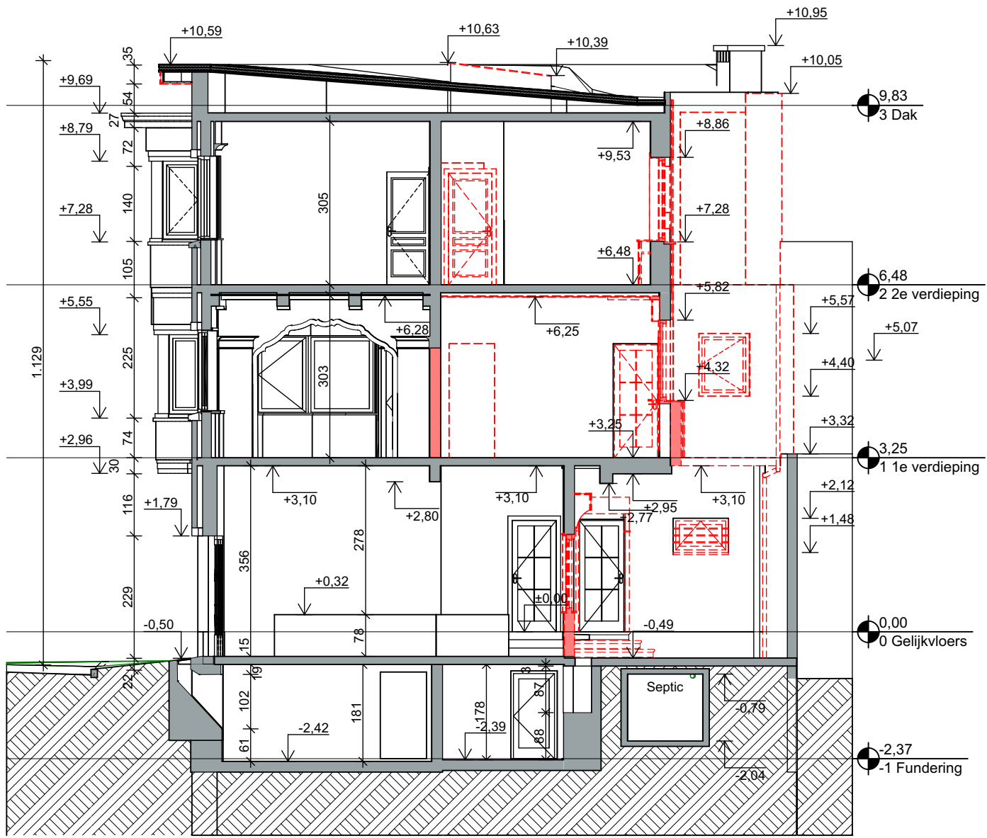
A Doorsnede A-A 1:100
