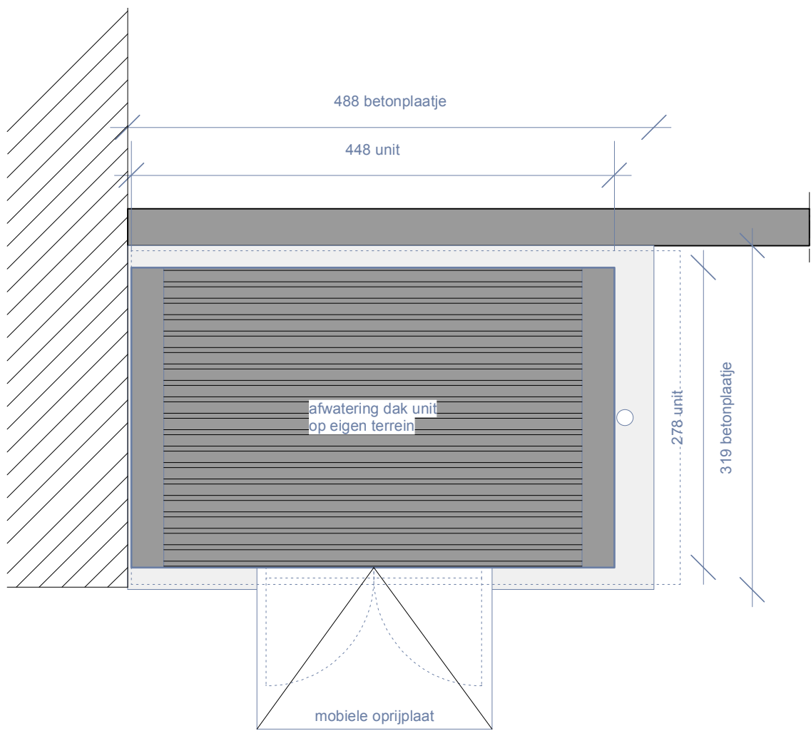
DAK PLAN SCHAAL 1/50
