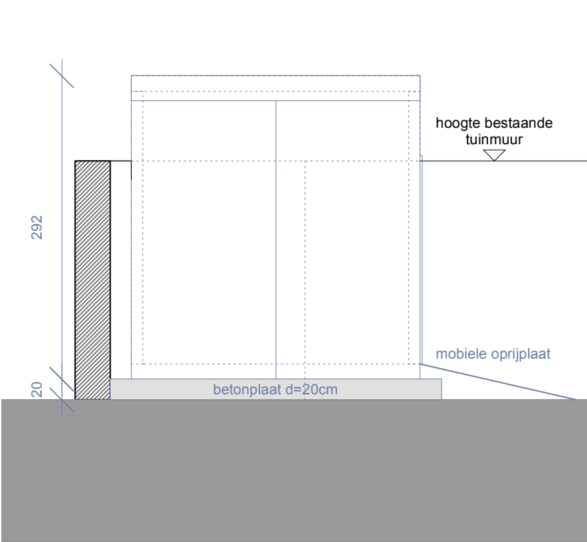
ZIJAANZICHT SCHAAL 1/50
