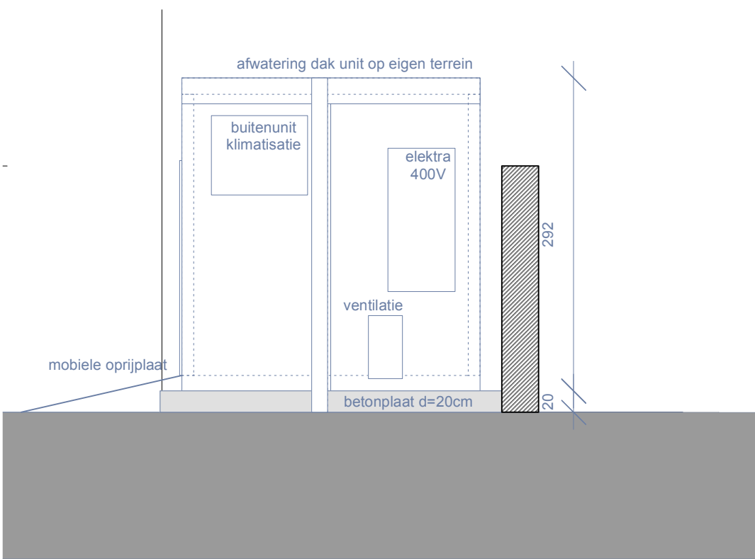
ZIJAANZICHT SCHAAL 1/50
