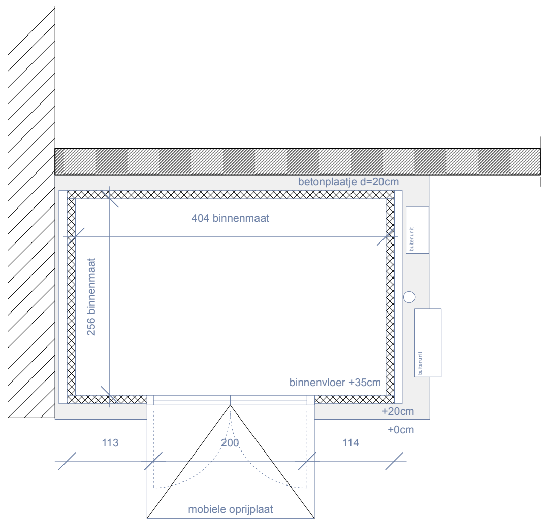
PLAN UNIT GELIJKVLOERS SCHAAL 1/50 TECHNISCH: ZIE PRODUCTBLAD PRODUCENT
