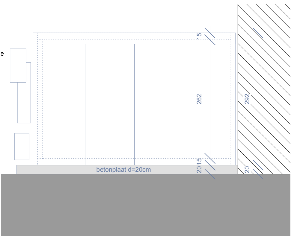
ACHTERAANZICHT SCHAAL 1/50
