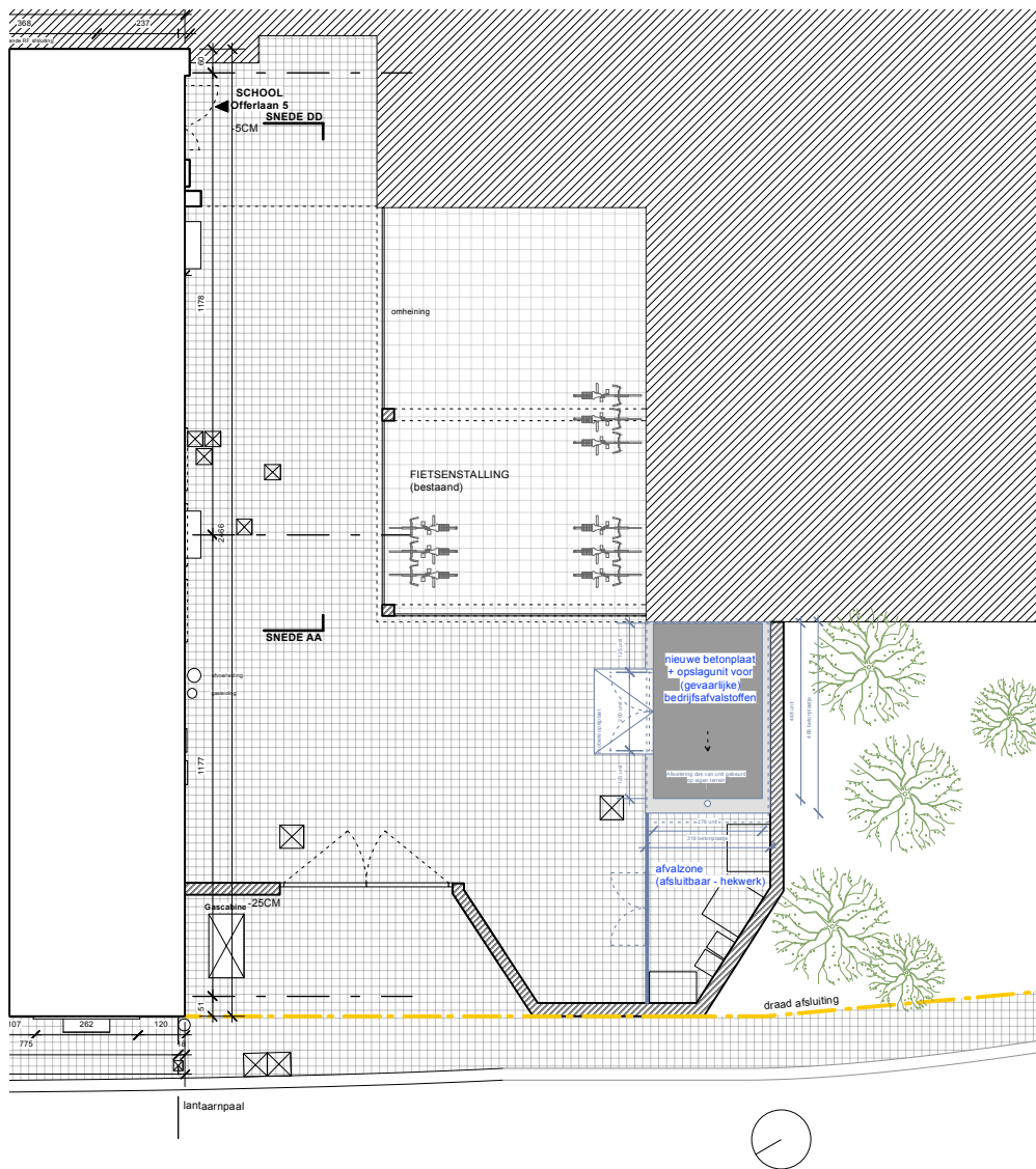
SITUERINGSPAN SCHAAL 1/200
