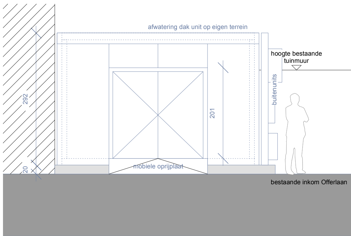
VOORAANZICHT SCHAAL 1/50
