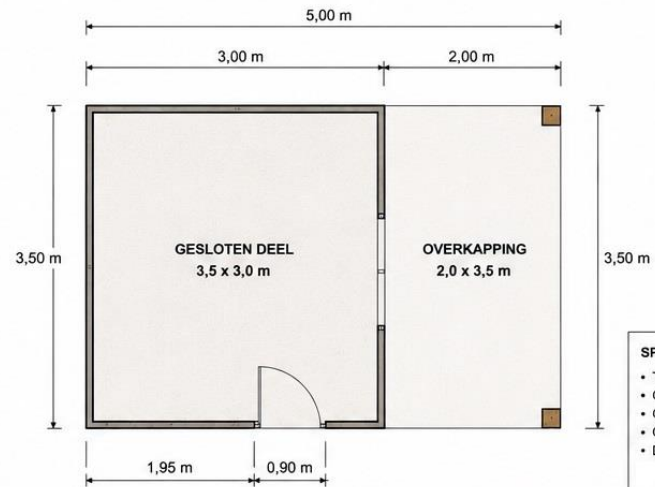
GRONDPLAN (bovenaanzicht)
