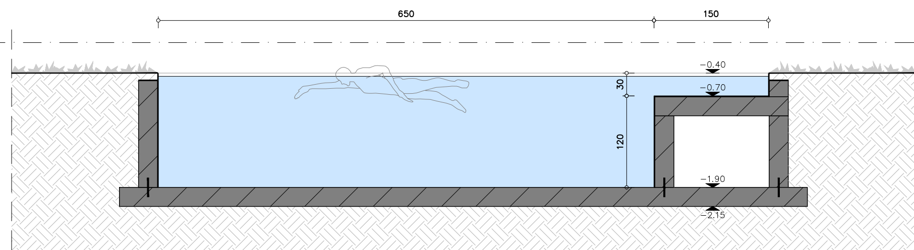
SNEDE BB'
