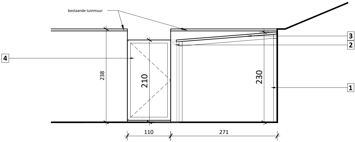
doorsnede - zijaanzicht
