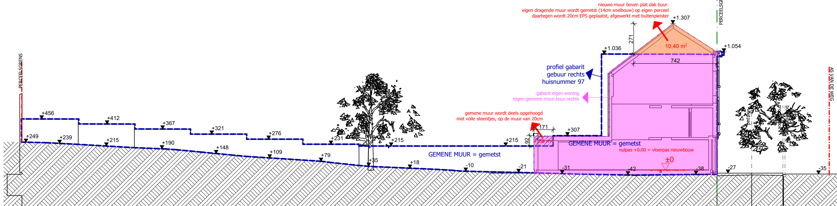
Terreinprofiel 2 - Nieuwe toestand
