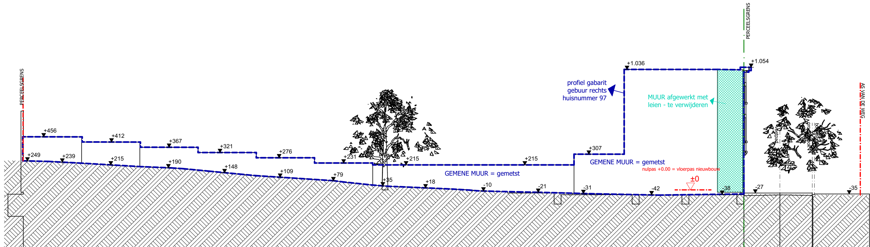
Terreinprofiel 2 - Bestaande toestand
