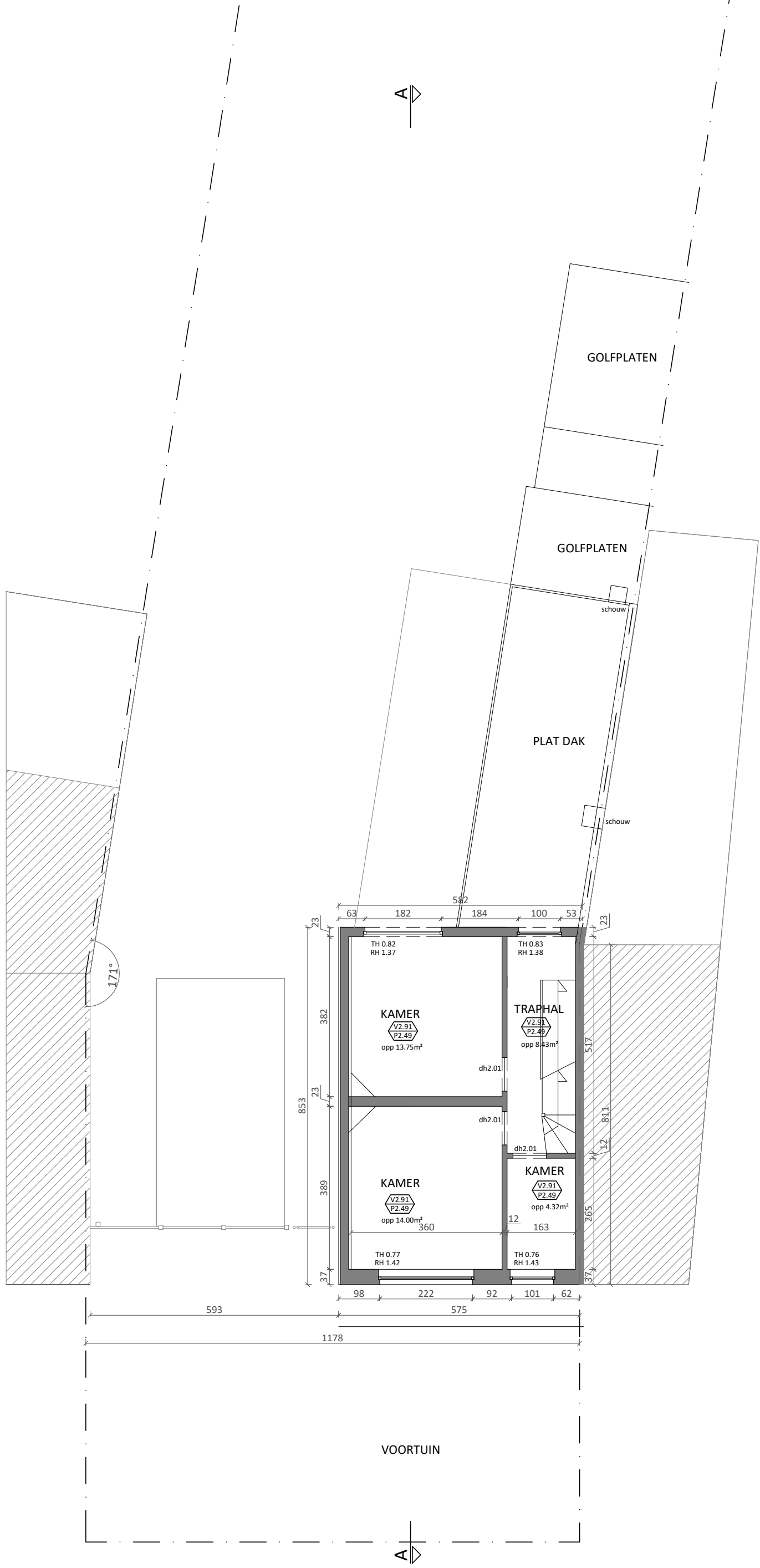
BESTAANDE TOESTAND EERSTE VERDIEPING schaal 1-100
