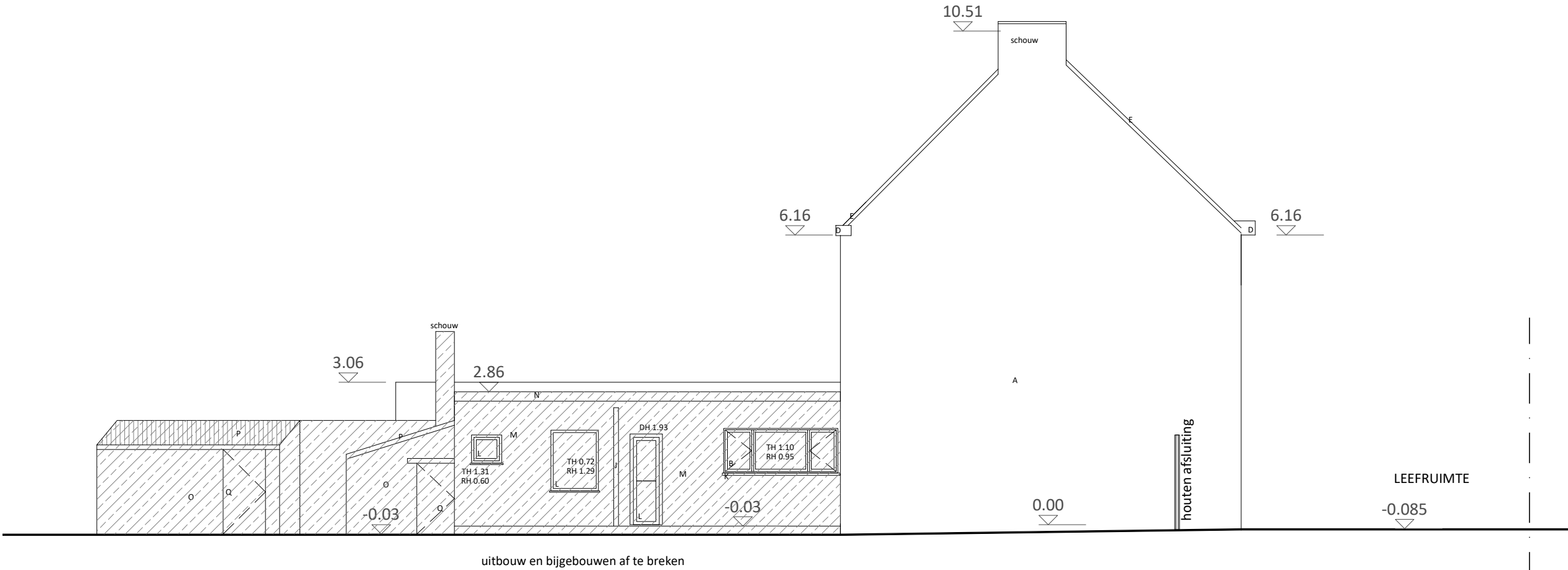
BESTAANDE TOESTAND ZIJGEVEL 1-100
