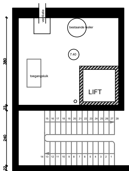
TUSSENVERDIEPING 1-2
