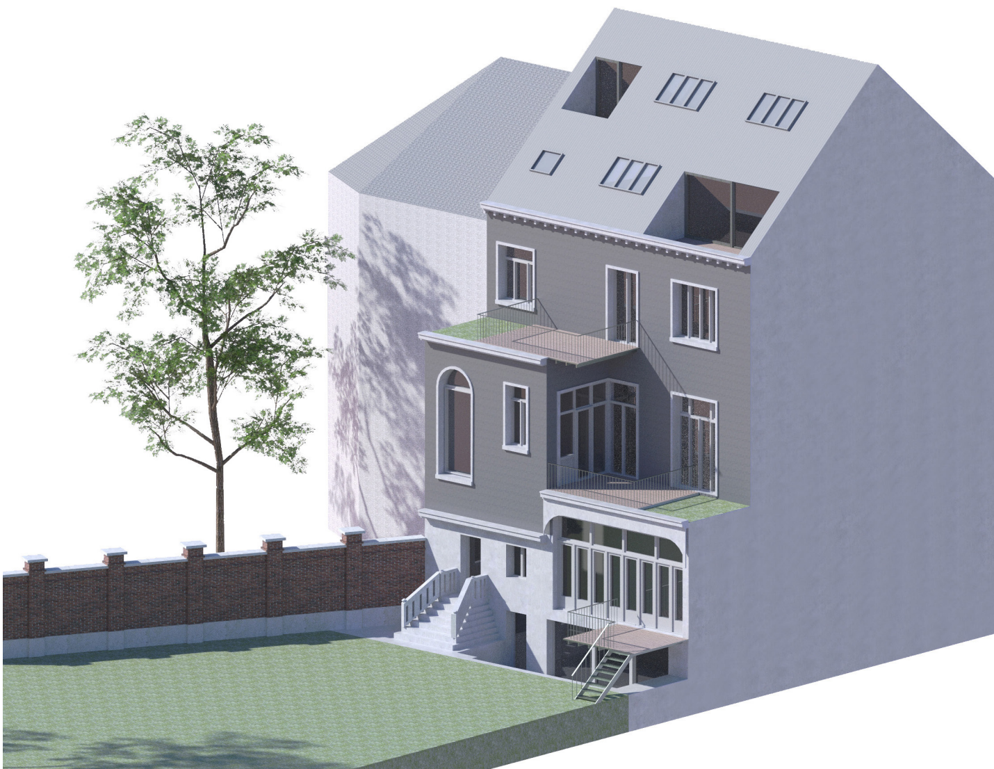
zicht van tuinzijde naar pand Kasteellaan (afstanden terrassen naar burens 1,9m)
