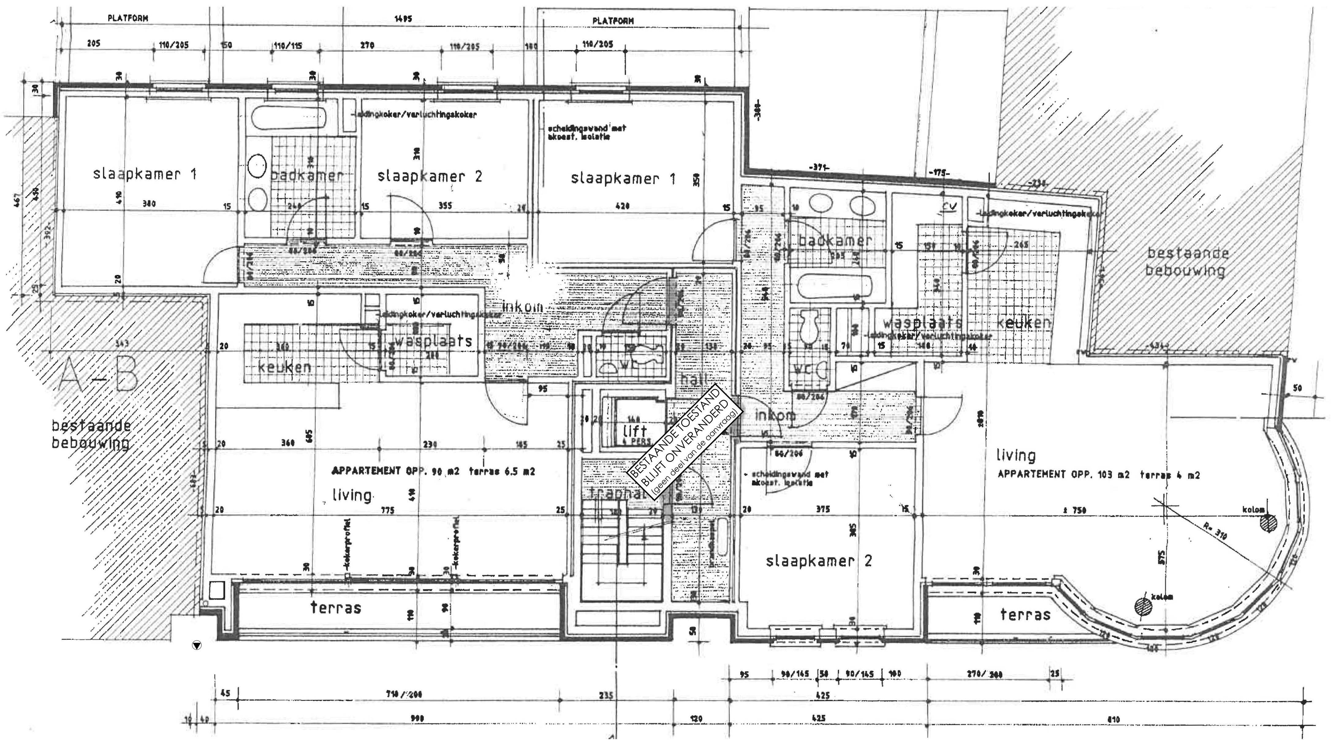
VERDIEPING 2 Bestaande toestand (volgens as-builtondossier)
