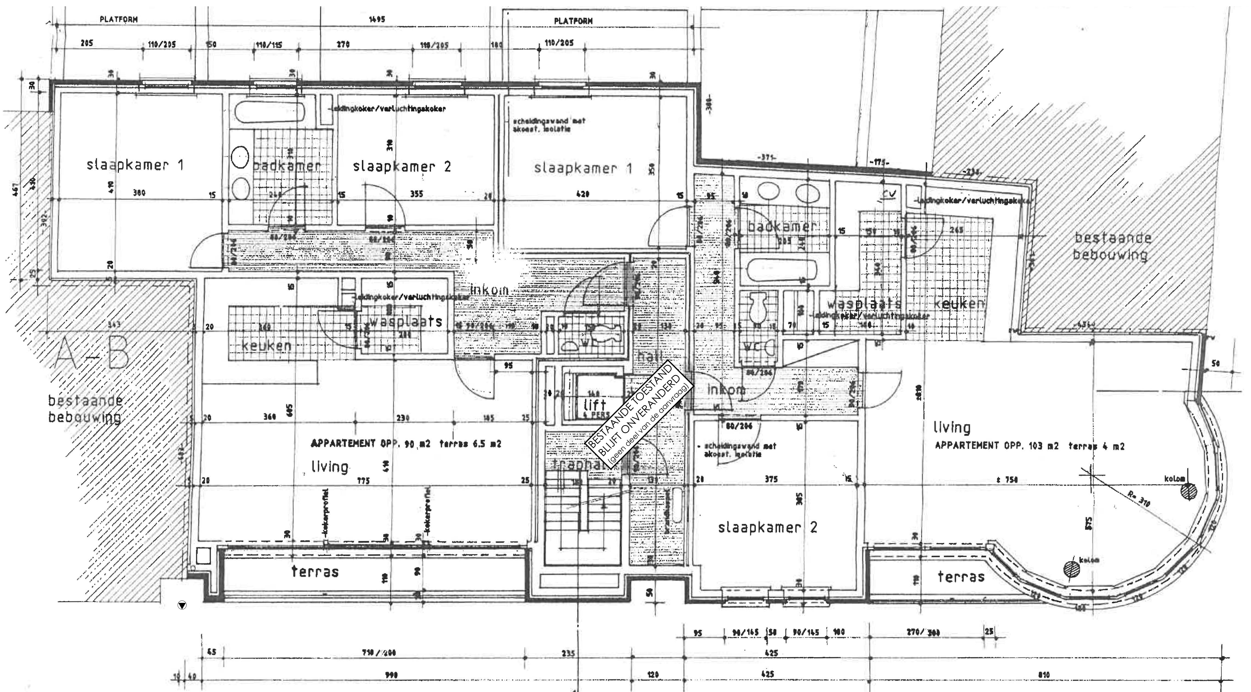
VERDIEPING 1 Bestaande toestand (volgens as-builtondossier)
