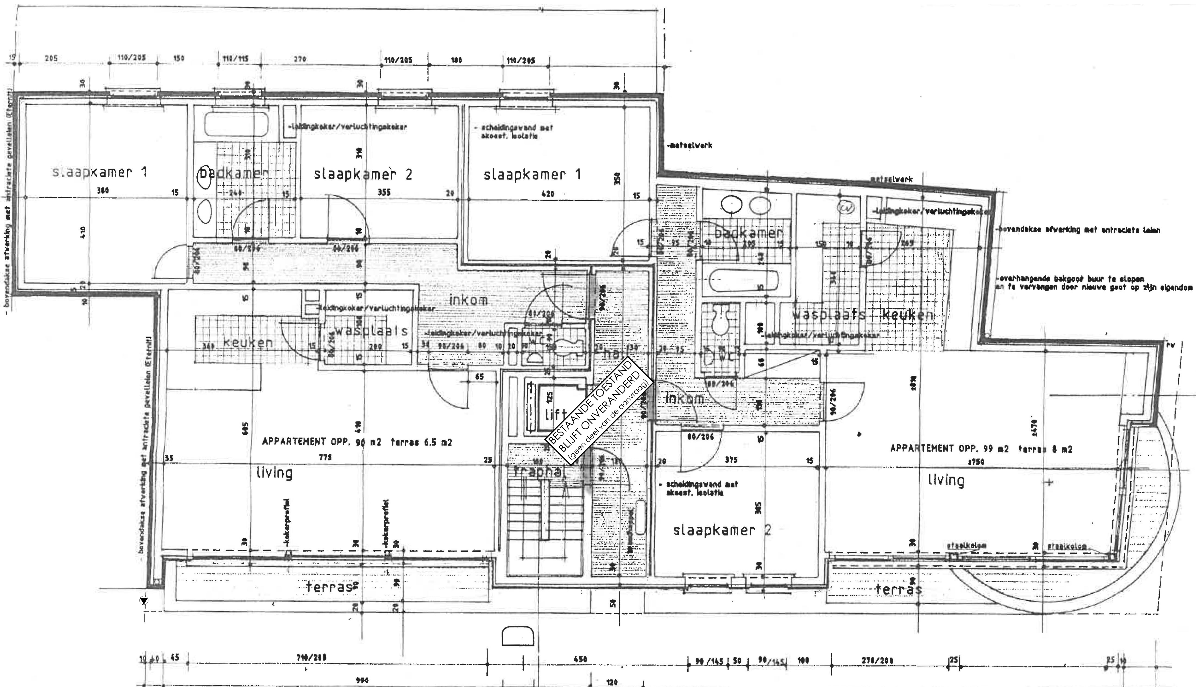
VERDIEPING 3 Bestaande toestand (volgens as-builtondossier)
