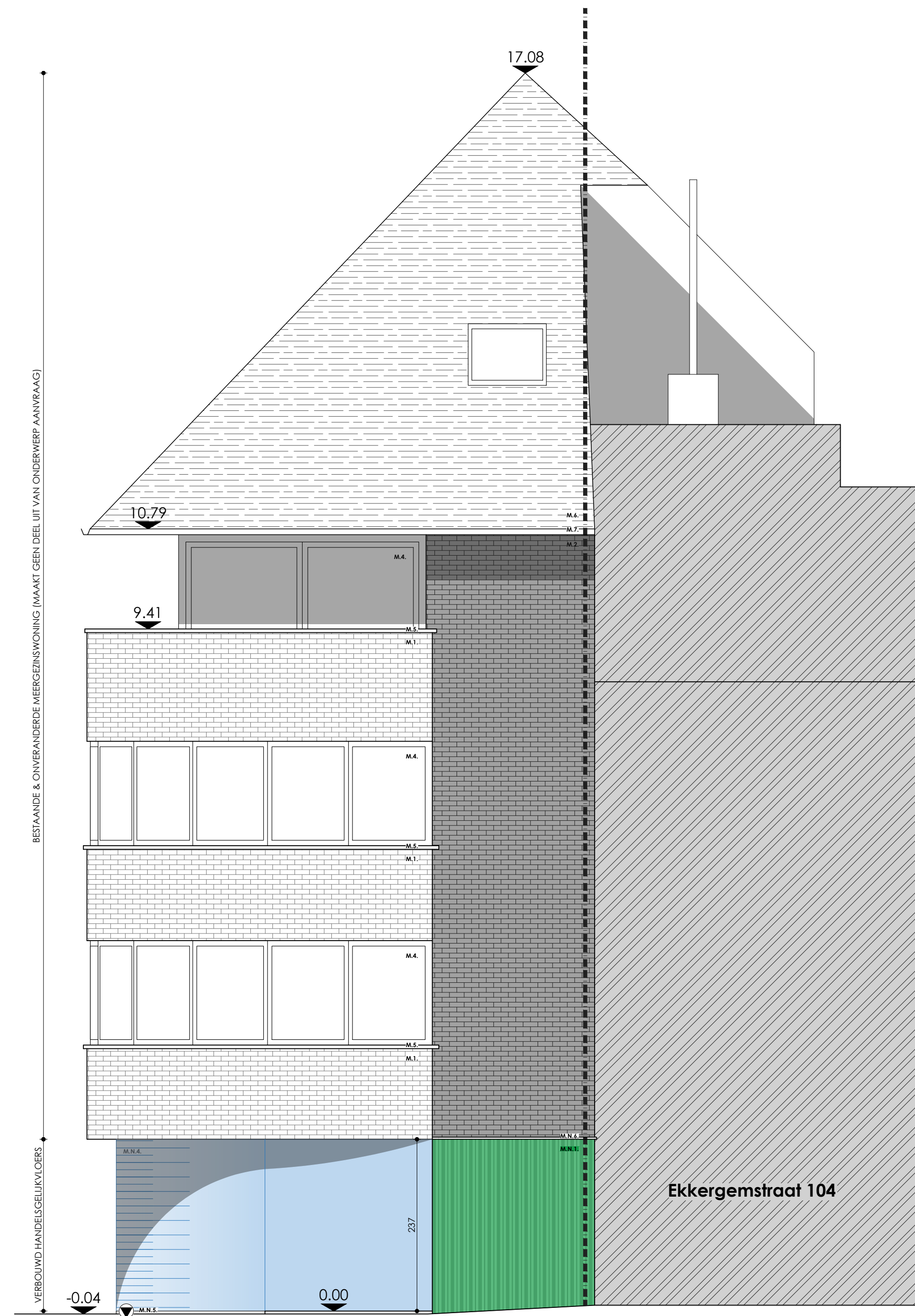
ZIJGEVEL RECHTS Nieuwe toestand
