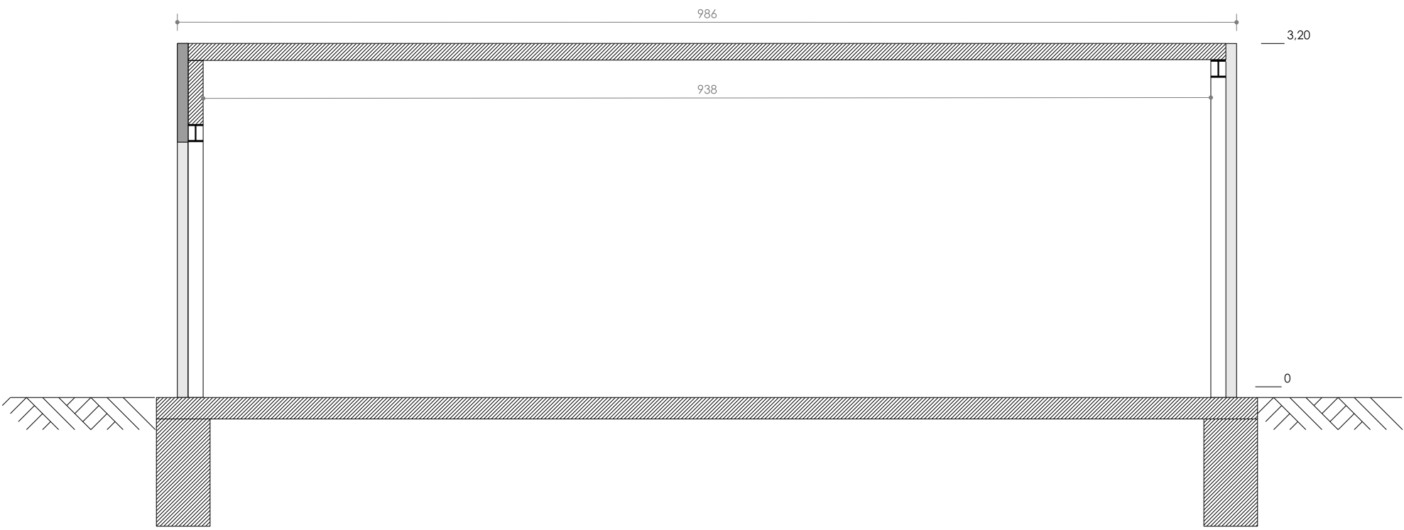
Garage snede
