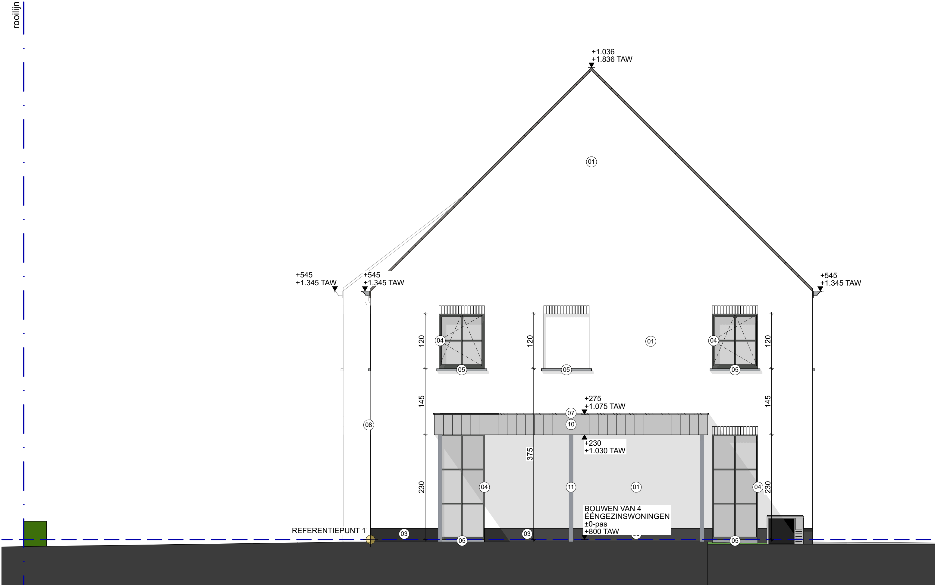
ZIJGEVEL RECHTS lot 16B schaal 1:50
