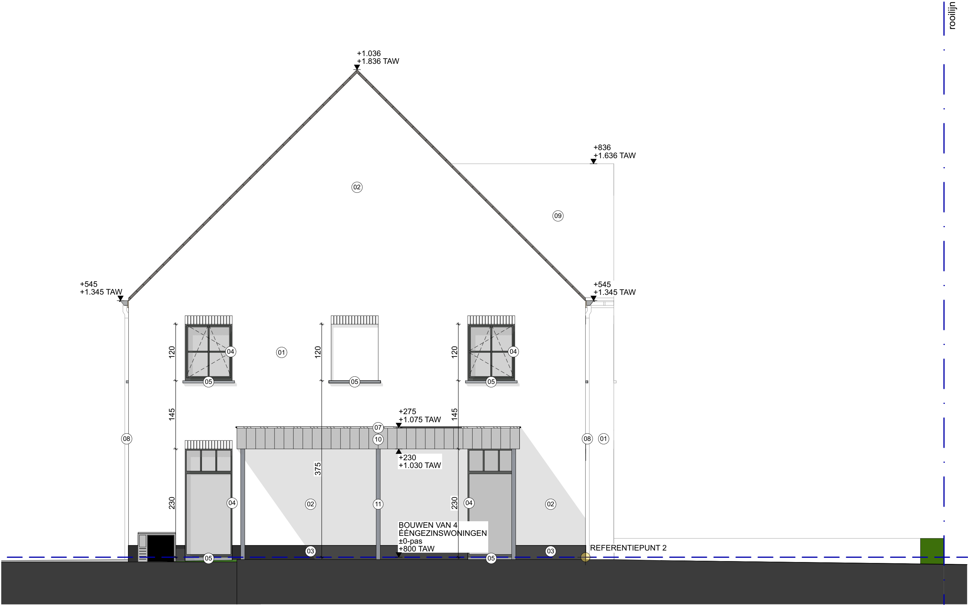
ZIJGEVEL LINKS lot 15A schaal 1:50 NIEUWE TOESTAND
