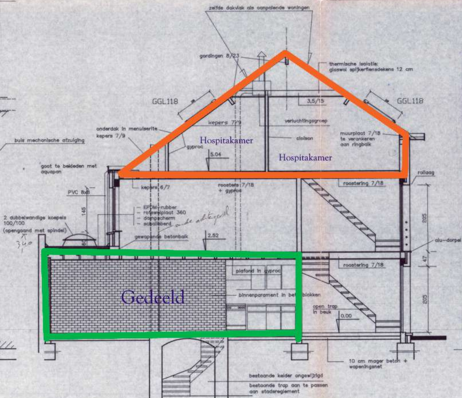
DOORSNEDE AA
