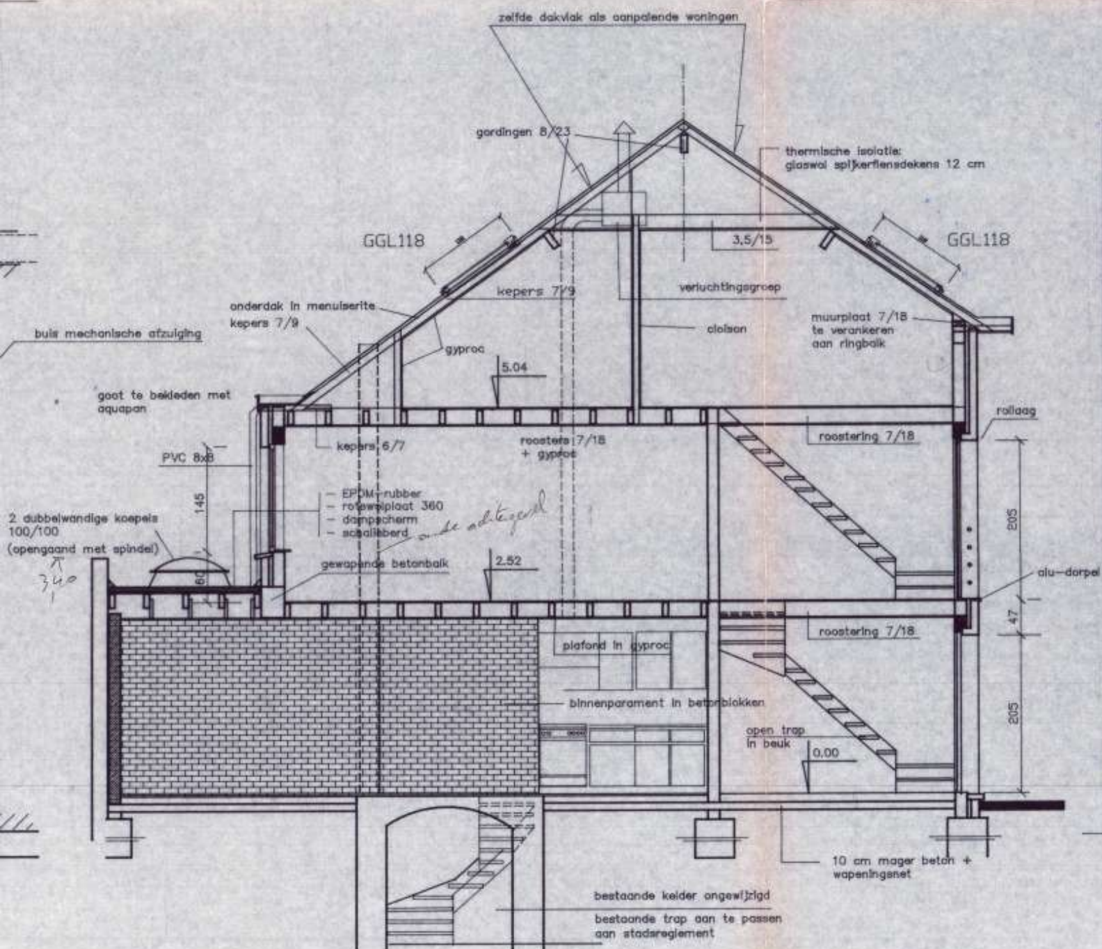
DOORSNEDE AA
