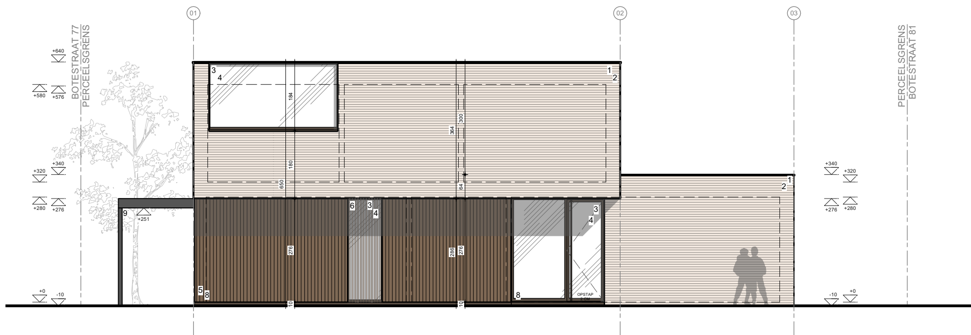
VOORGEVEL - NOORD
