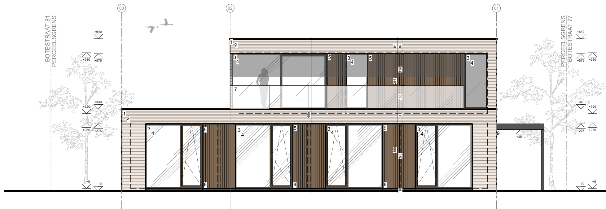
ACHTERGEVEL - ZUID
