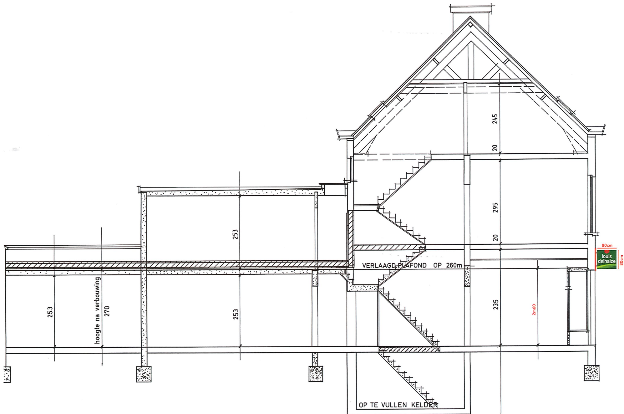
DOORSNEDE : HUIDIGE SITUATIE
