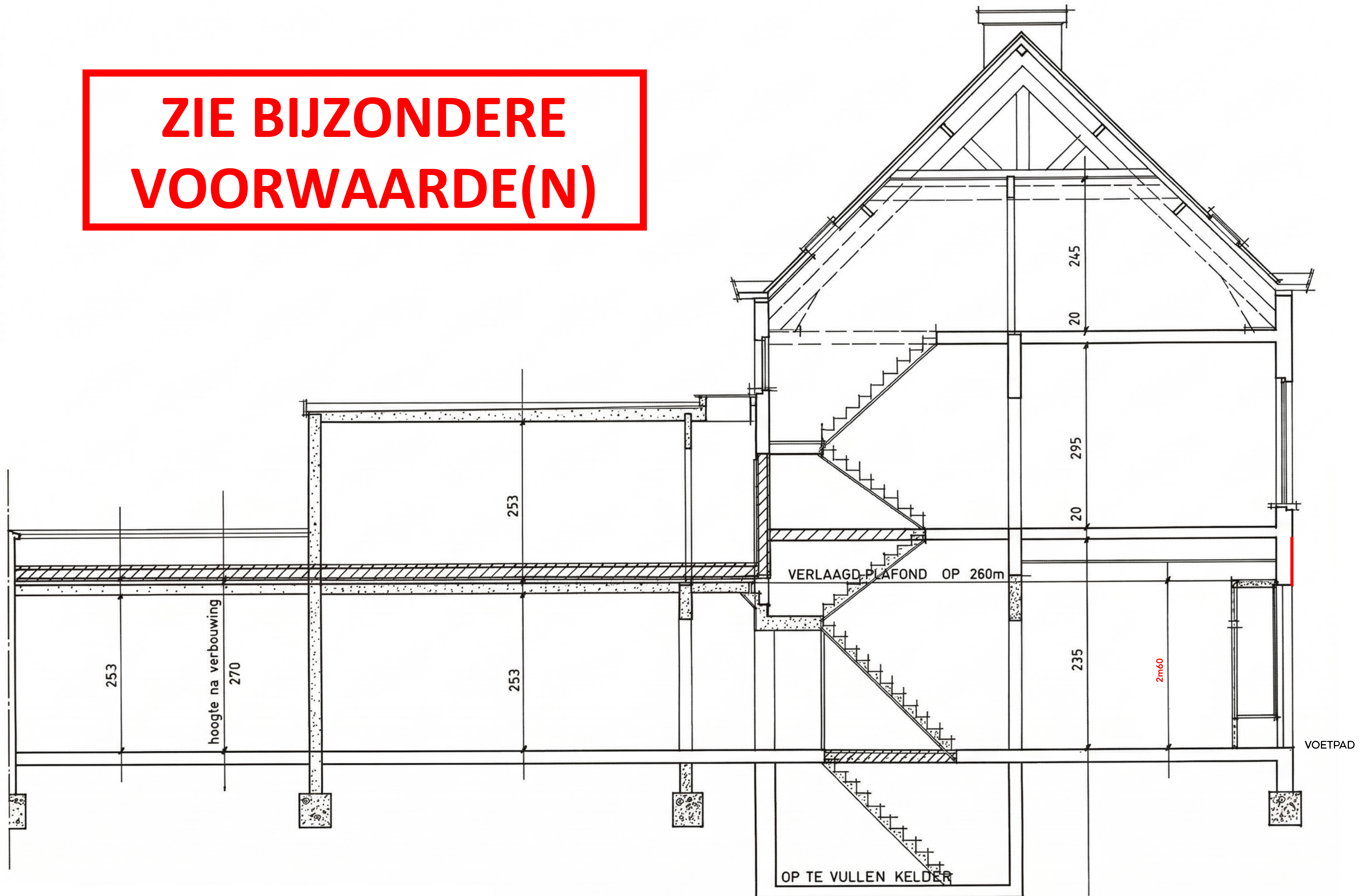
DOORSNEDE : TOEKOMSTIGE SITUATIE
