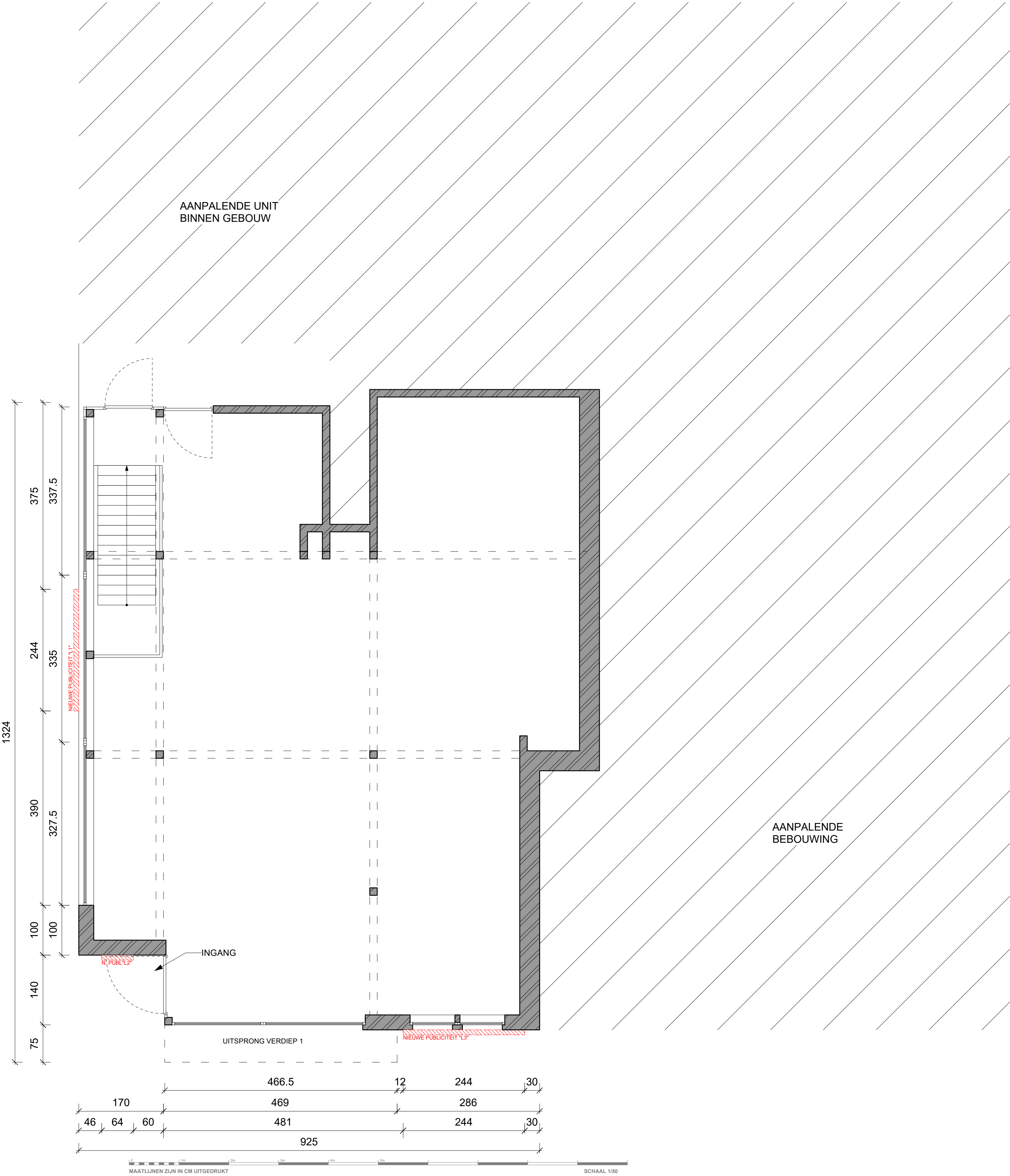
GRONDPLAN-GELIJKVLOERS NIEUWE TOESTAND
