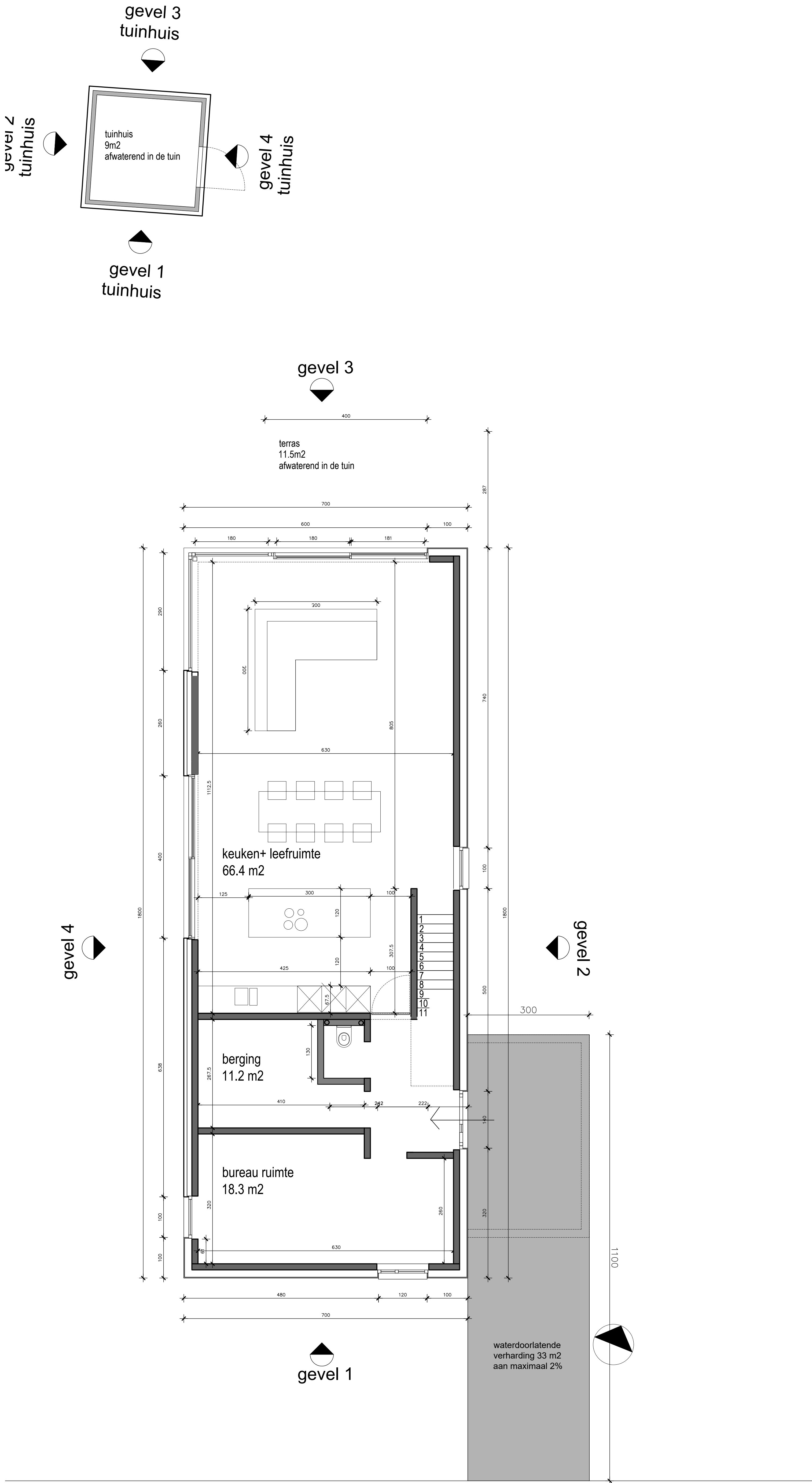
GRONDPLAN gelijkvloers nieuwe toestand scenario 1 schaal: 1/50
