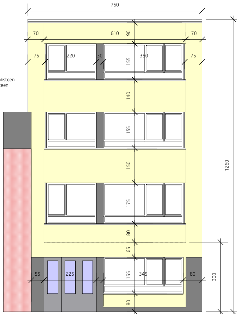
VOORGEVEL _ BESTAANDE TOESTAND 1/100
