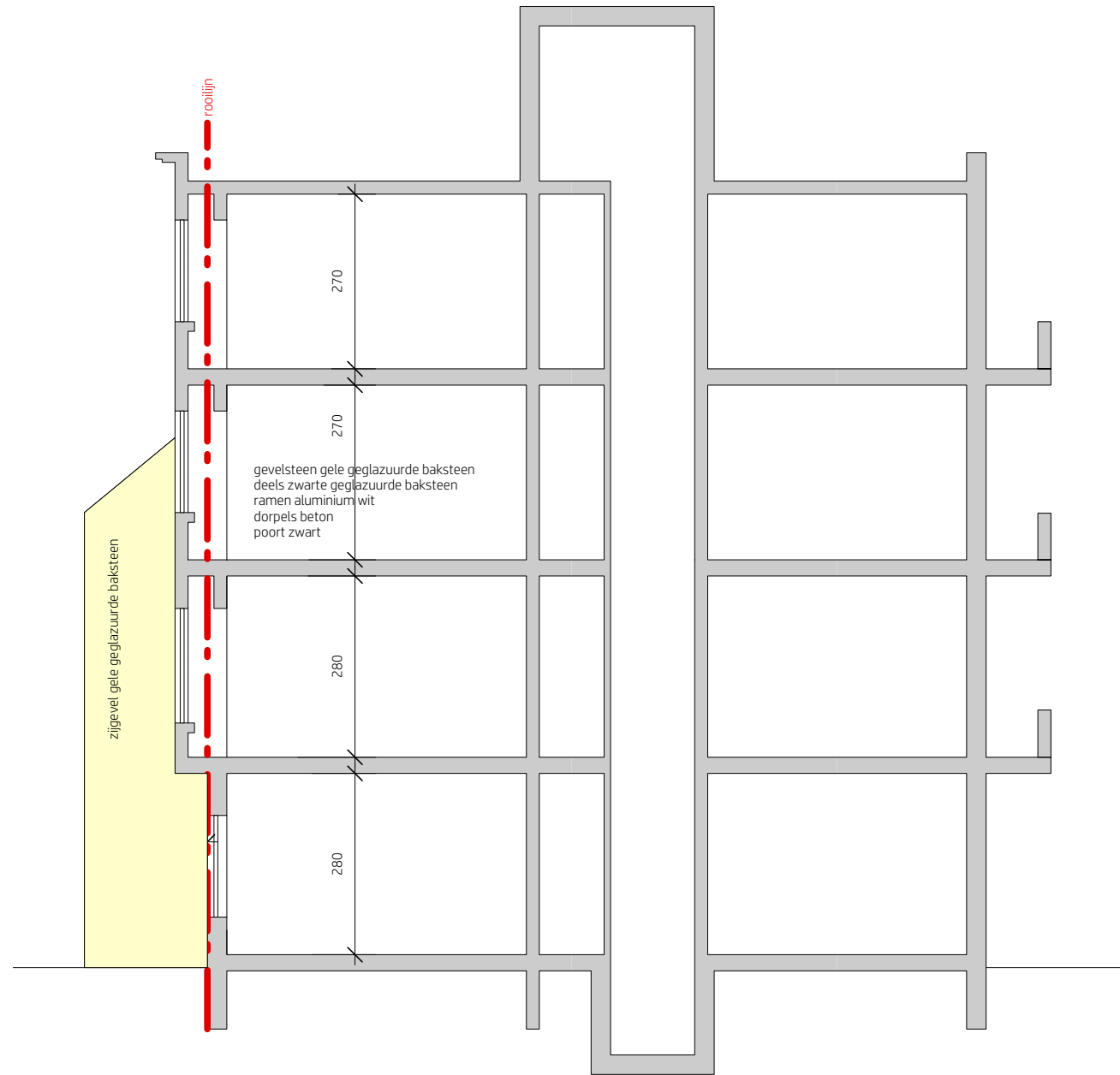
SNEDE _ BESTAANDE TOESTAND 1/100
